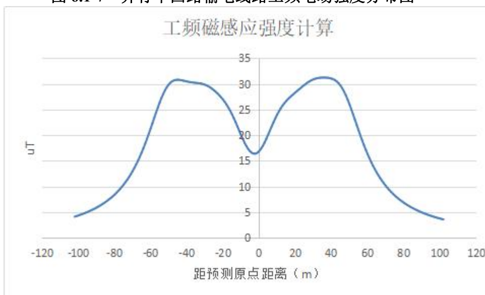
图 6.1-8 并行单回路输电线路工频磁感应强度分布图
