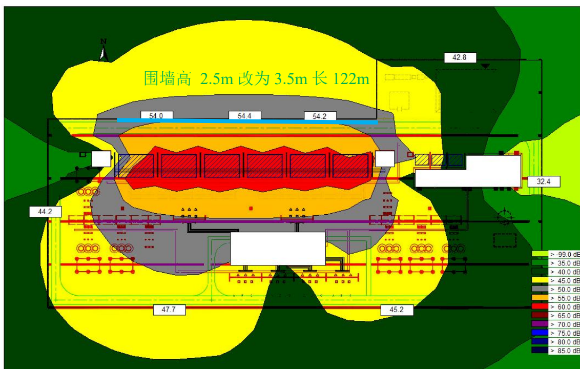
图 6.2-3 汇集站声源设备采取措施后噪声预测等效 A 声级图
