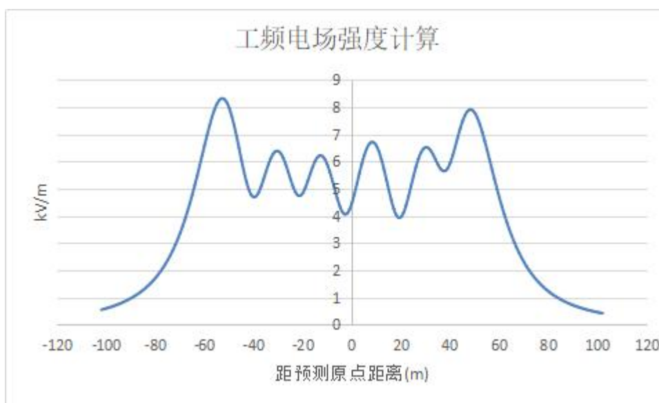
图 6.1-7 并行单回路输电线路工频电场强度分布图
