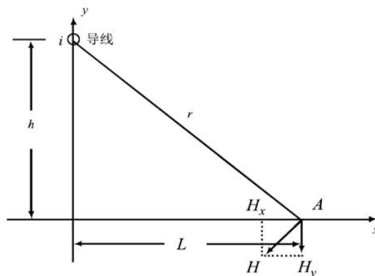
图 6.1-5 磁场向量图
