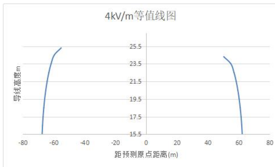
图 6.1-9 并行单回路输电线路 4kV/m 等值线图
