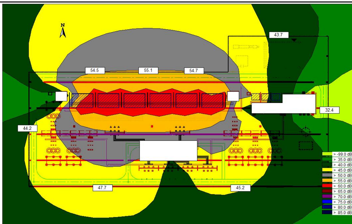
图 6.2-2 汇集站声源设备采取措施前噪声预测等效 A 声级图
