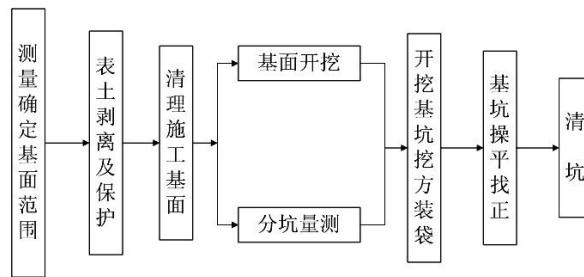
图 3.1-1 基坑开挖施工工艺流程图
