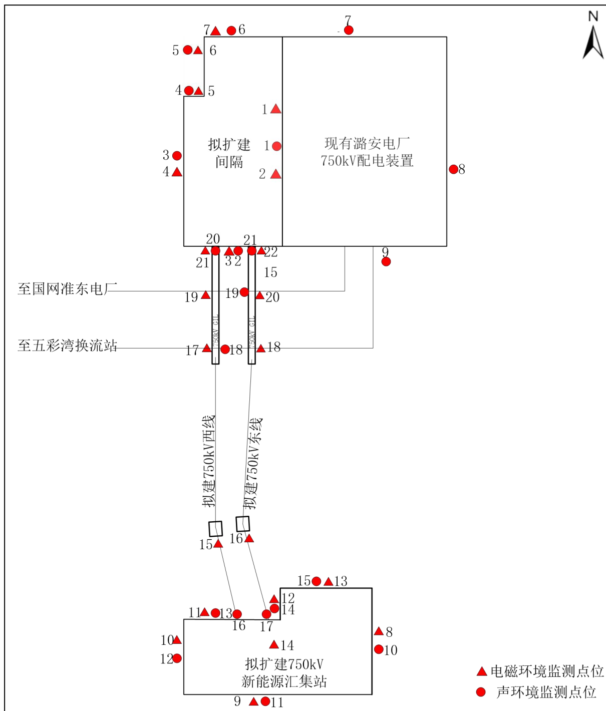
图 4.2-1 工频电磁场及噪声现状监测分布图
