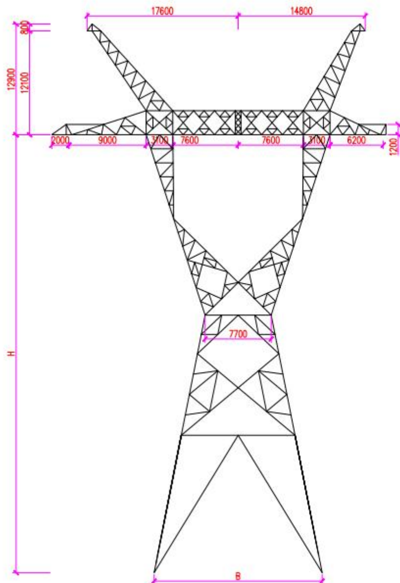
图 6.1-6 并行单回路电磁理论预测典型塔型
