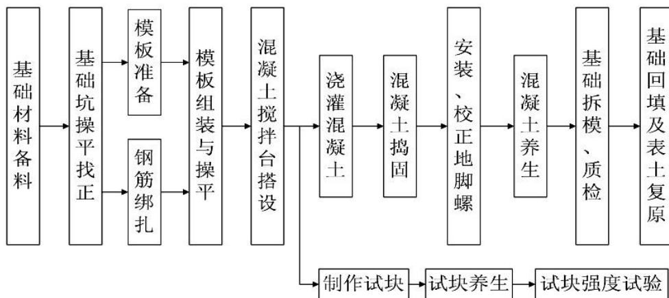
图 3.1-2 基础施工工艺流程图
