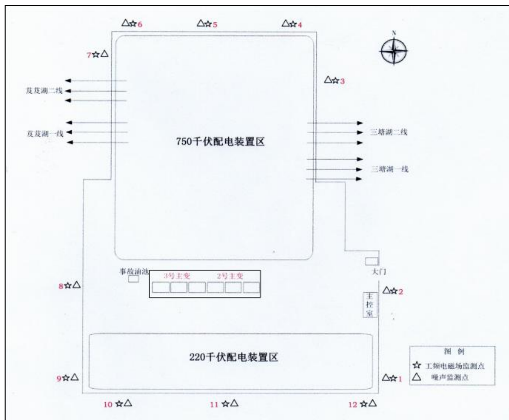
图 6.1-1 类比项目监测布点图
