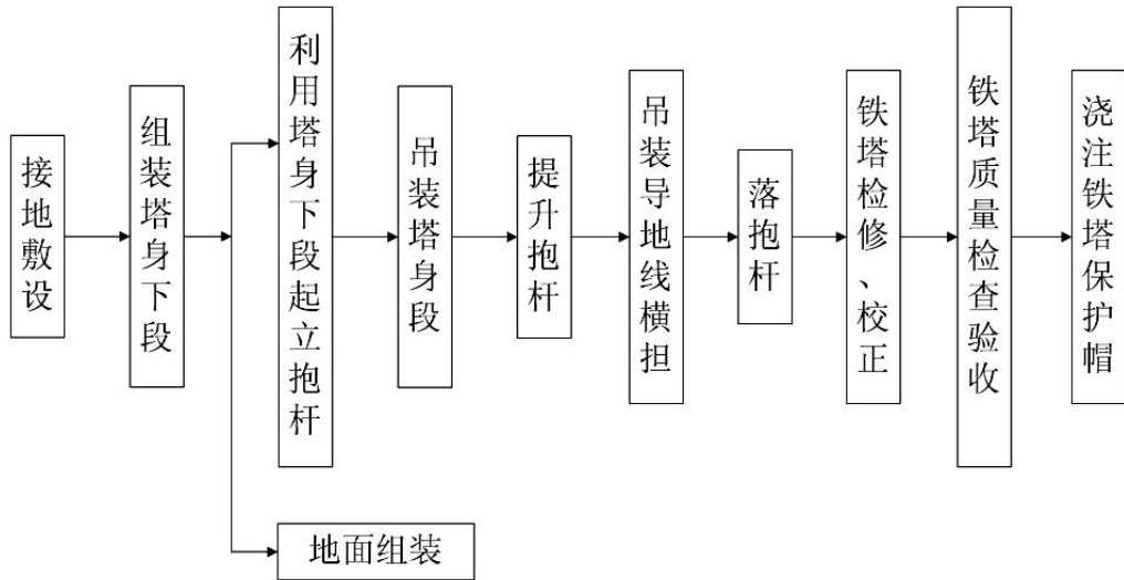
图 3.1-3 铁塔组立接地施工工艺流程图
