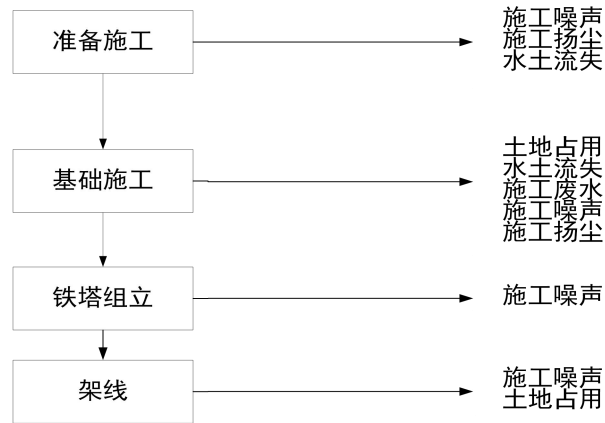
图 3.3-2 输电线路施工工艺及产污环节
