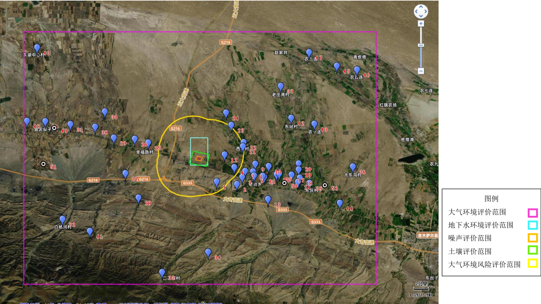
图2.8.2-1 评价范围与敏感目标分布图
