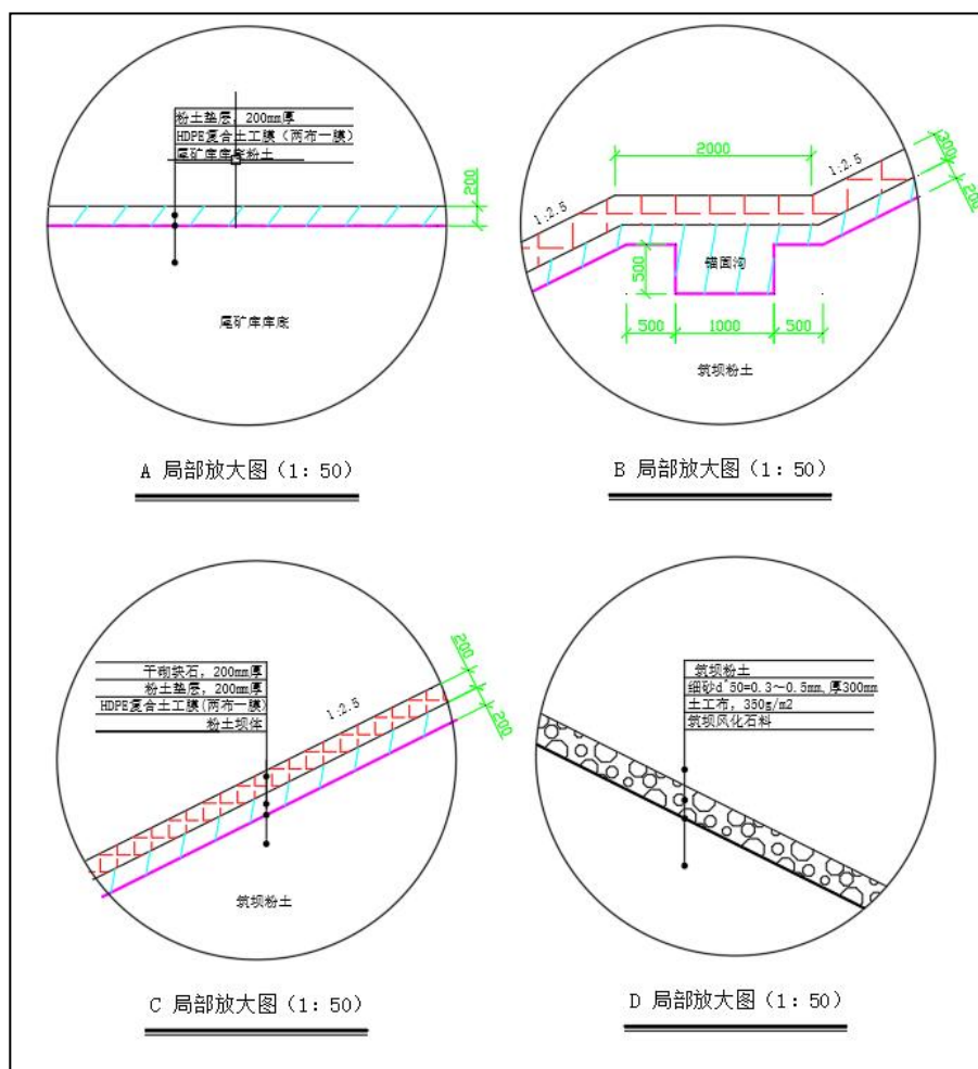
图 3.1-4 尾矿库防渗剖面图
