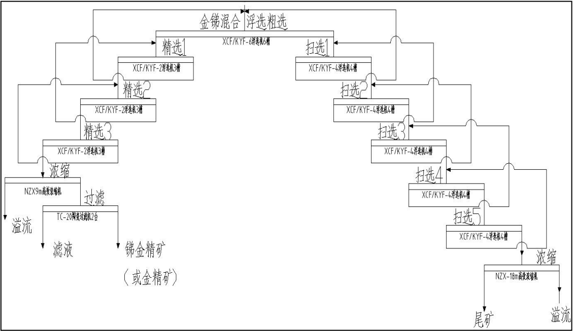
图 3.1-3 浮选、浓缩、过滤流程图
