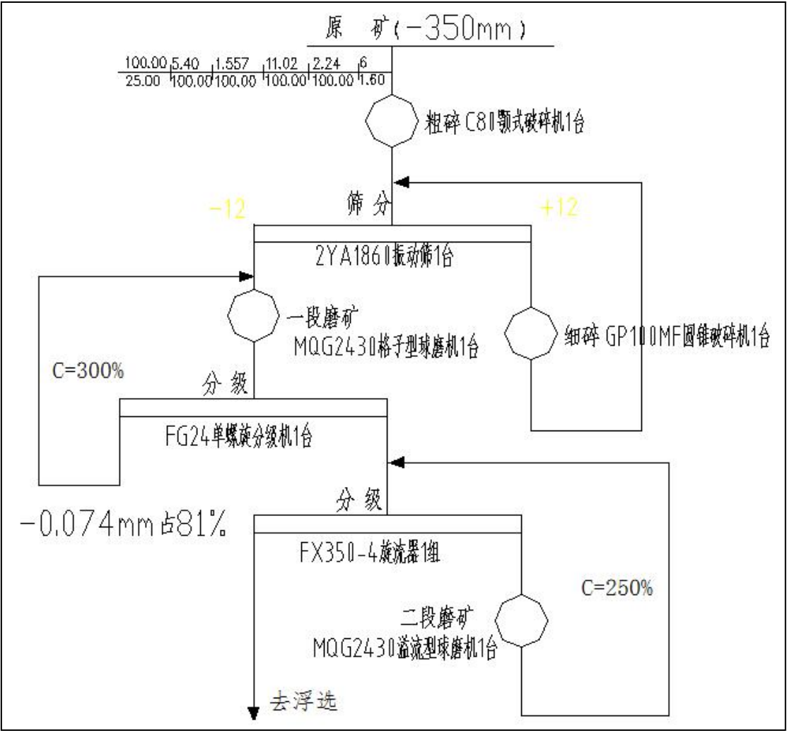
图 3.1-2 破碎磨矿流程图
