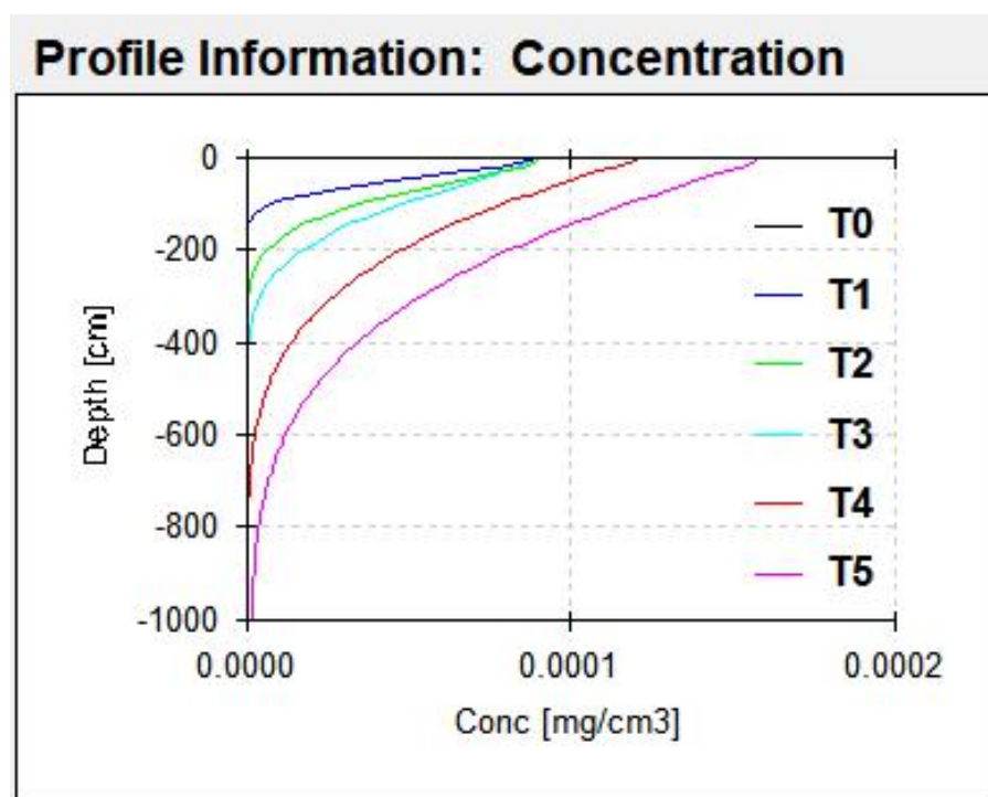
图 5.2-6 汞运移预测结果
