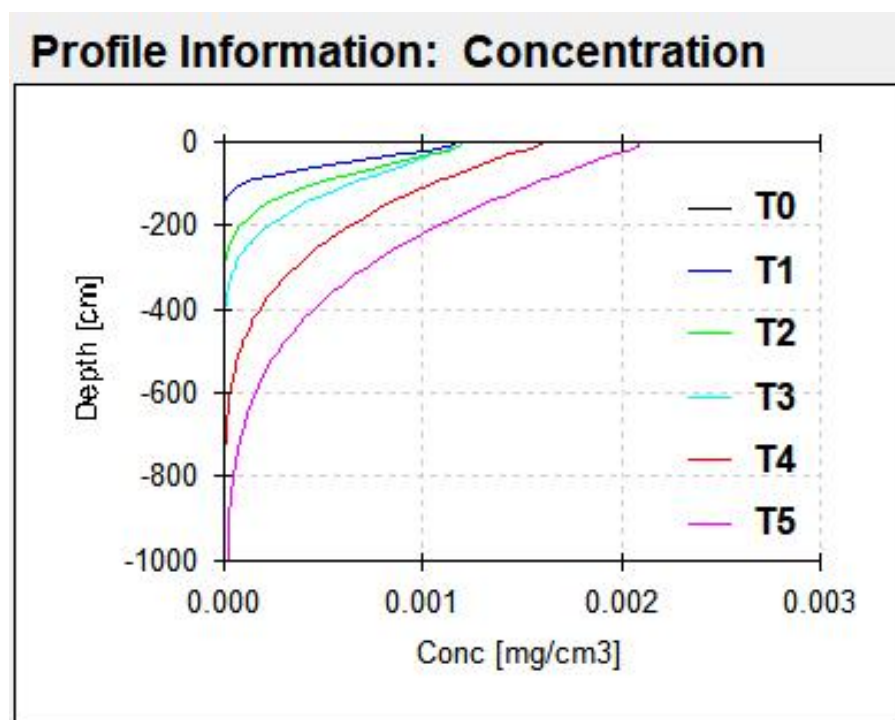
图 5.2-7 砷运移预测结果
