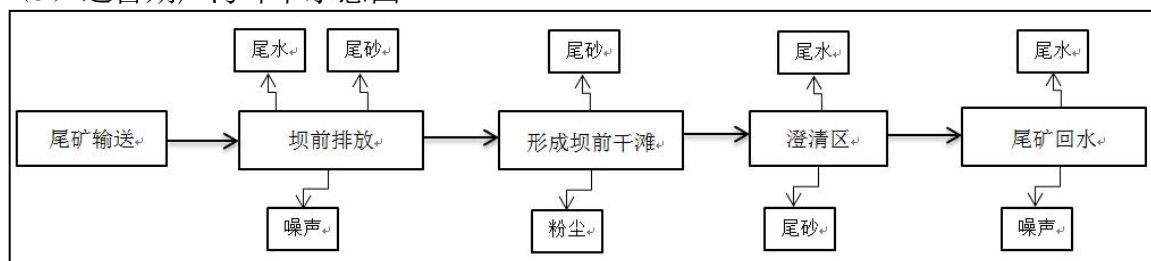
图 3.2-4 运营期产污环节示意图
