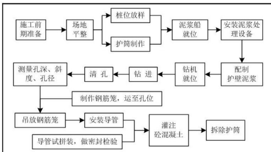
图 3.5-3 钻孔灌注桩基础施工工艺流程图
