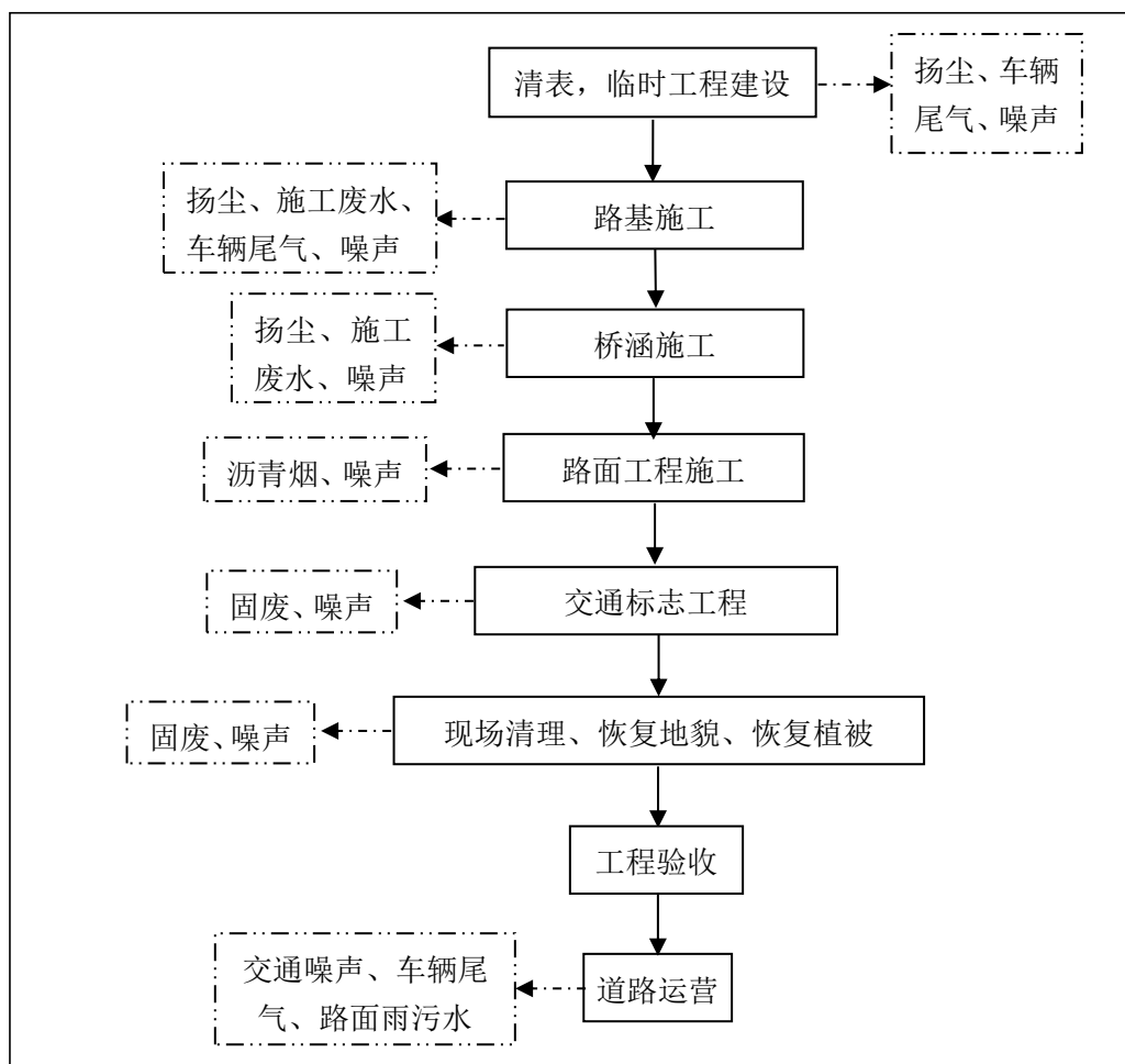
图 3.5-1 道路施工工艺流程图
