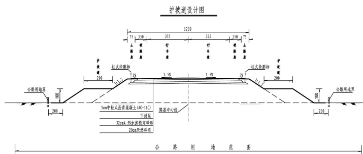
图 3.3-7 本项目道路护道坡设计示意图
