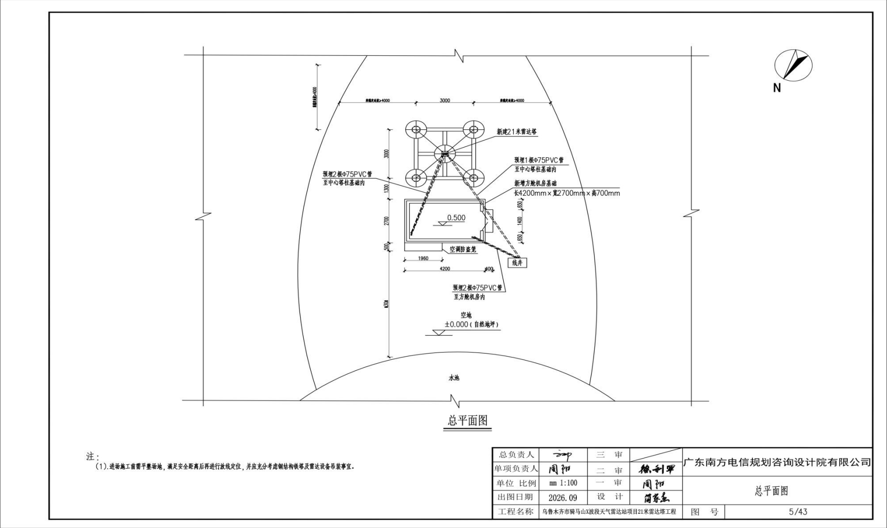
附图 2 本项目施工图纸
