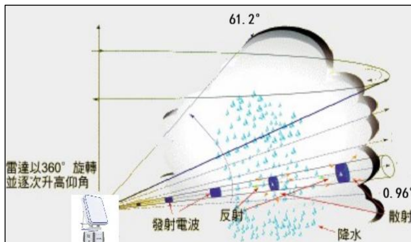
图 2-4 X 波段相控阵气象雷达系统工作原理图
