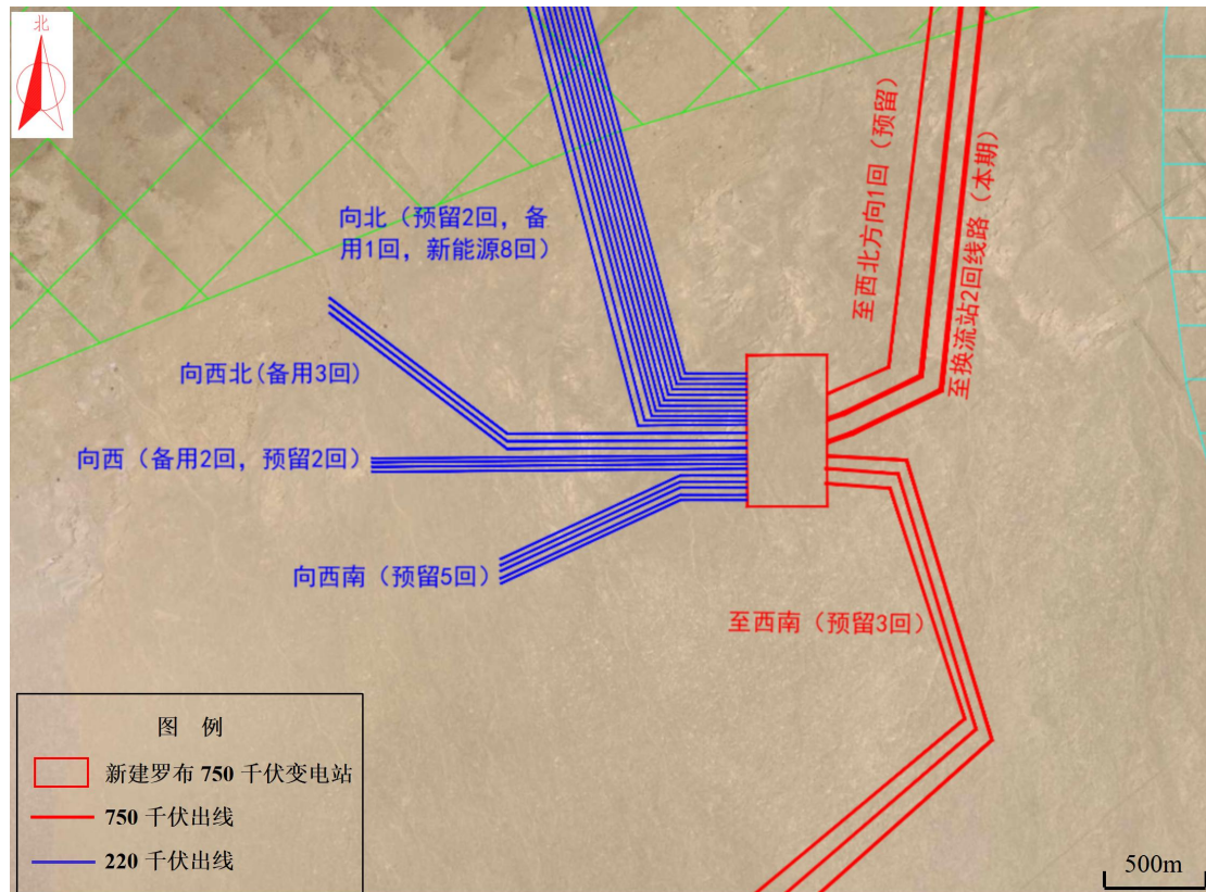
图 3.1-2 罗布 750 千伏变电站出线示意图
