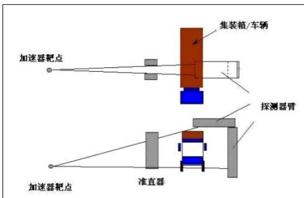
图 9-2 MB1215DE (BX) 系统 X 射线透射成像系统示意图
