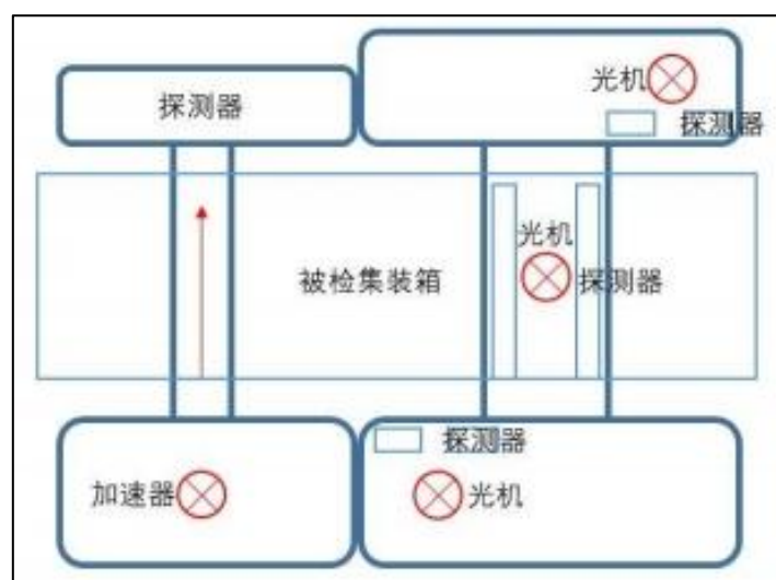
图 9-4 设备构成示意图
