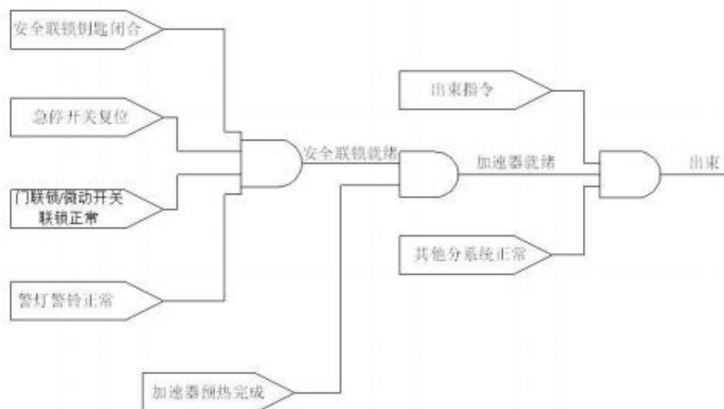
图 10-3 电子加速器系统安全联锁逻辑示意图
