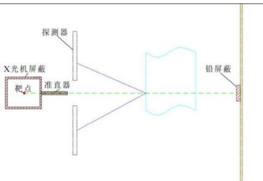
图 10-2 MB1215DE（BX）系统屏蔽示意图
