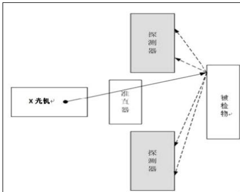
图 9-3 MB1215DE (BX) 系统 X 射线背散射成像系统示意图
