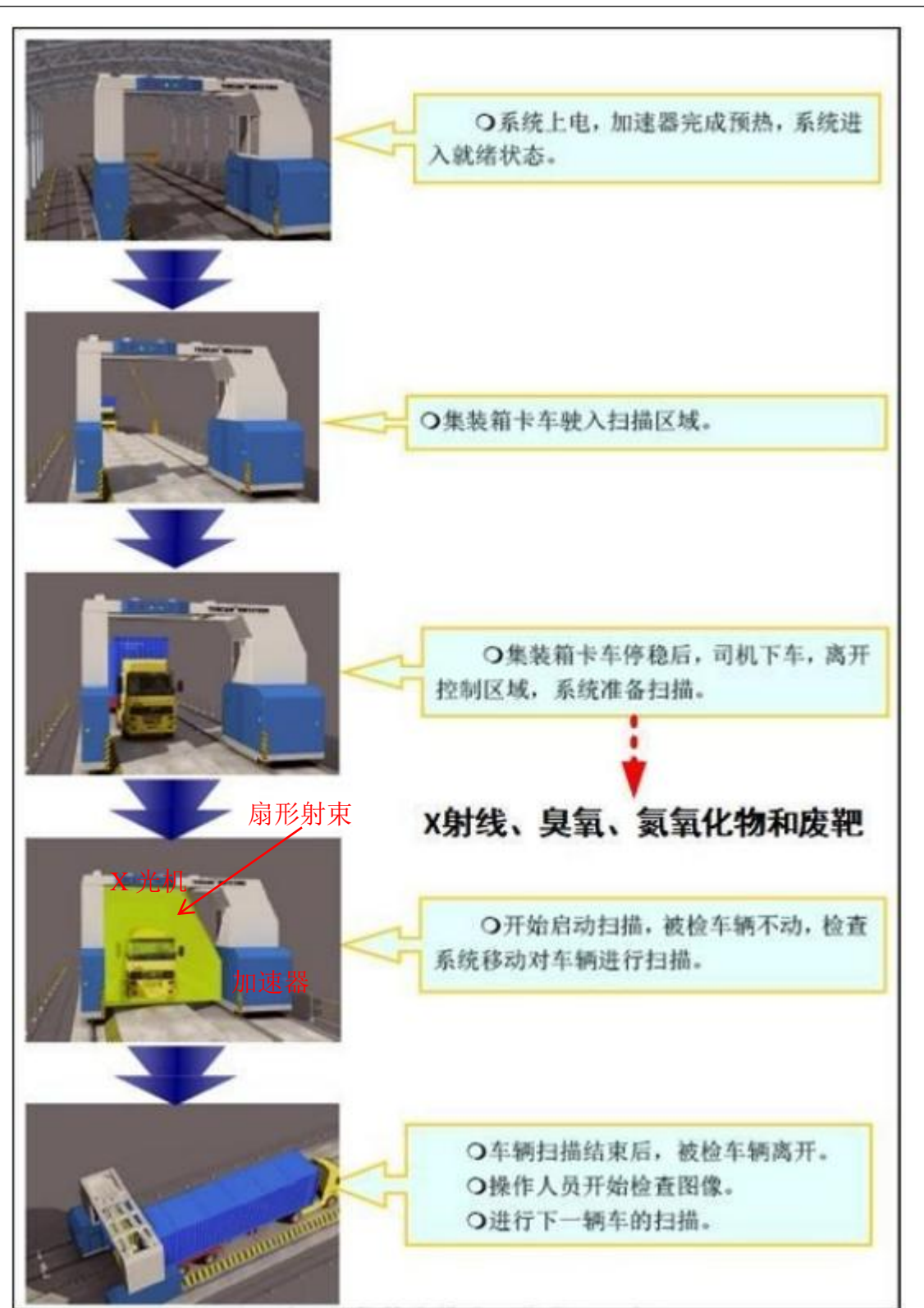
图 9-7 同类型集装箱/车辆检查系统精细检查模式下的工作流程及产污示意图
