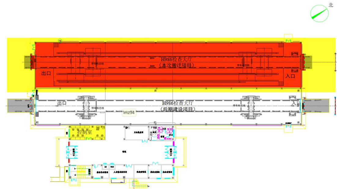
图 10-1 工作场所分区示意图（红色部分为控制区，黄色部分为监督区）
