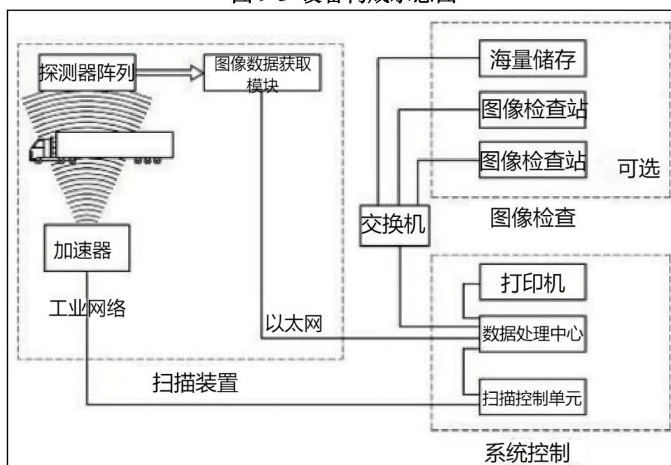
图 9-6 X 射线成像分系统示意图
