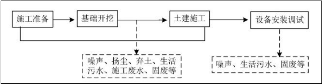
图3-3 施工期工艺流程及产污环节
