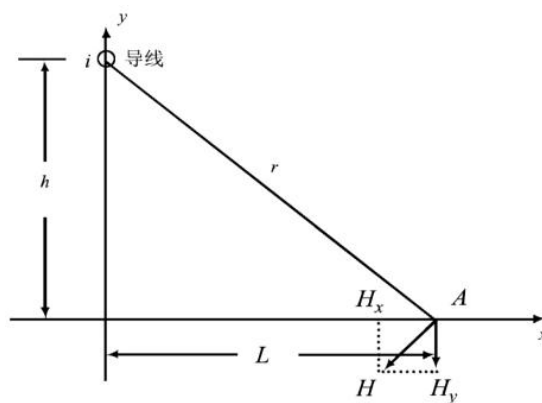
图 6.1-7 磁场向量图
