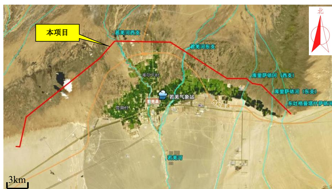
图 4.1-1 本项目输电线路跨越地表水位置示意图
