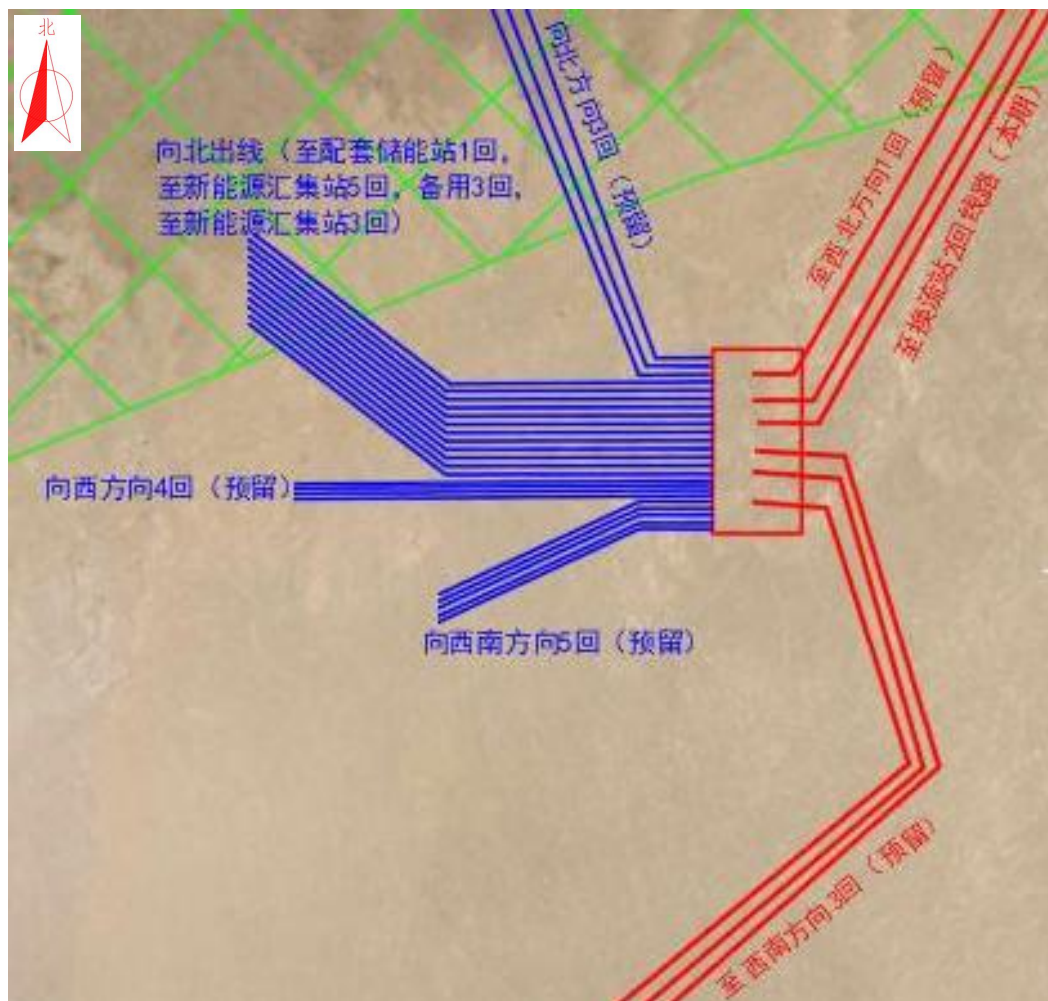
图 3.1-2 罗布 750 千伏变电站出线示意图
