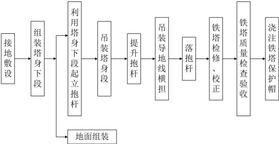
图 3.1-8 铁塔组立接地施工工艺流程图
