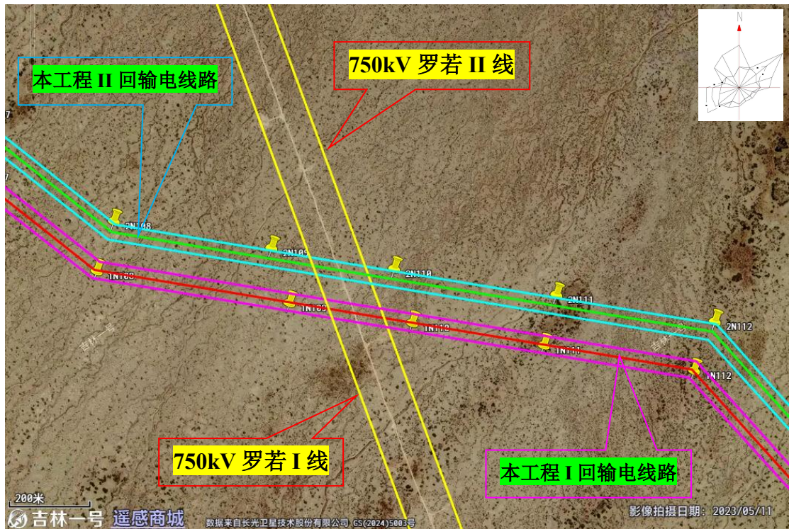
图 6.1-13 本工程输电线路跨越 750kV 罗若 I、II 线处示意图
