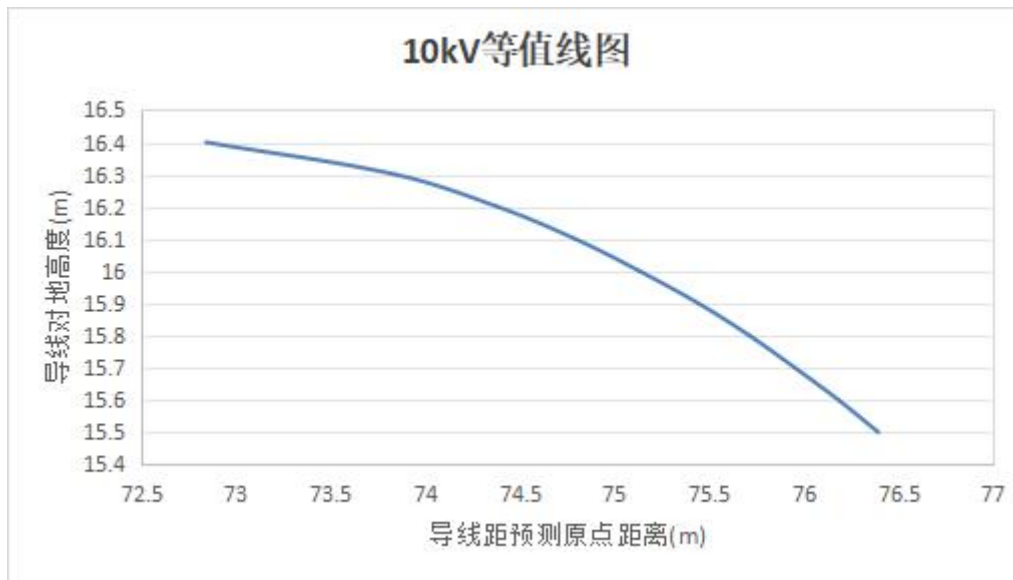
图 6.1-12 并行单回路输电线路 10kV/m 等值线图
