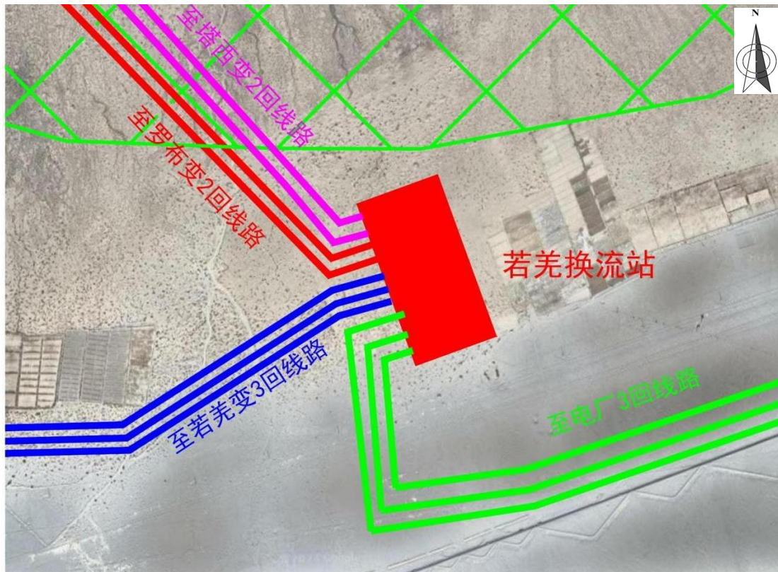
图 3.1-1 若羌换流站 750kV 出线示意图
