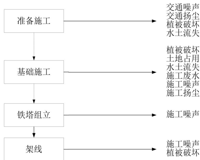
图 3.3-2 输电线路施工工艺及产污环节
