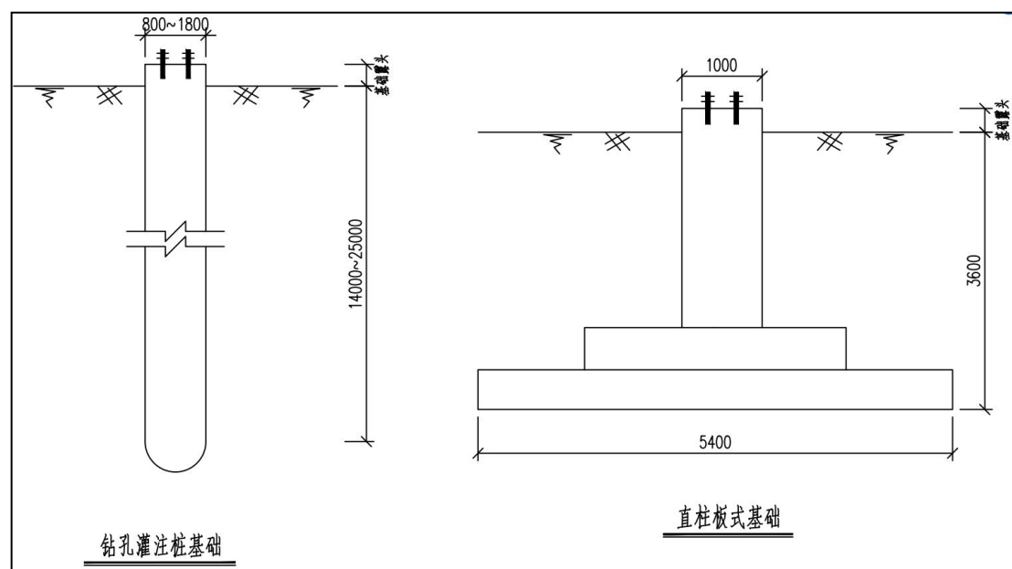
图 3.1-5 基础一览图
