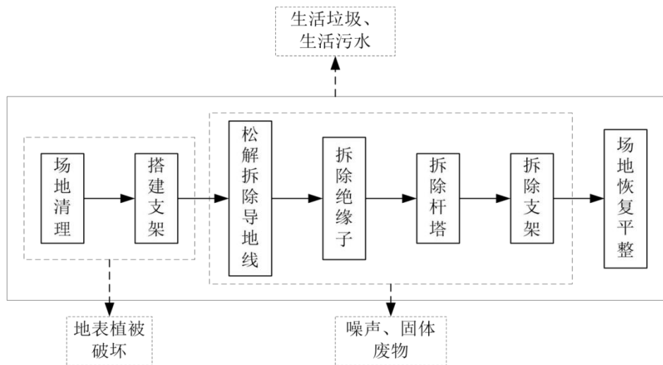
图 3.3-3 拆除既有输电线路施工工艺及产污环节 3.3.1.2运行期环境影响因素
