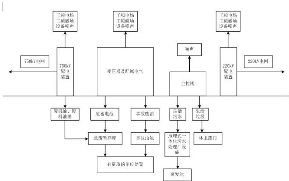
图 3.3-4 变电站运行期工艺流程及产污节点图 （2）输电线路工程
