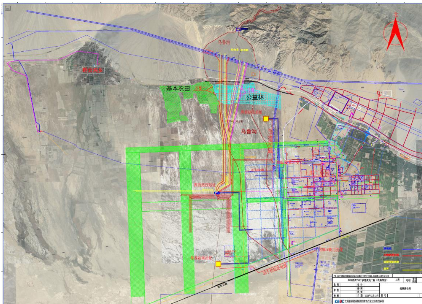
图 3.1-4 输电线路路径图
