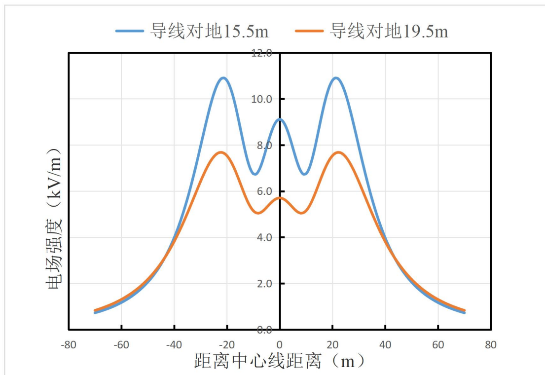
图 6.1-6 750kV 单回路输电线路工频电场强度分布图
