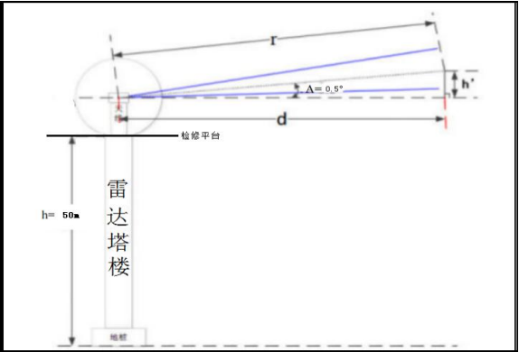
图 4-1 天线前方限高计算示意图
