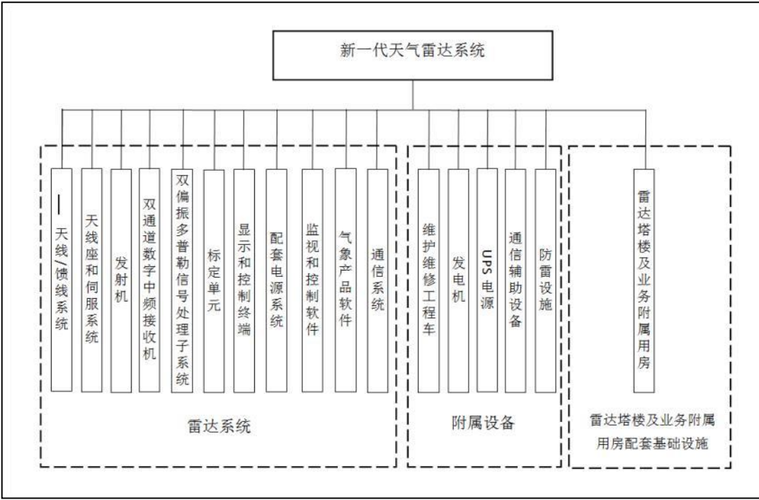
图 2-4 C 波段气象雷达系统组成示意图
