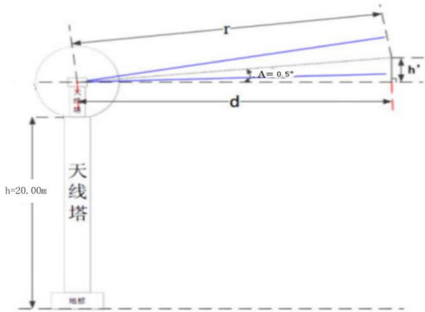
图6-1 天线前方限高计算示意图
