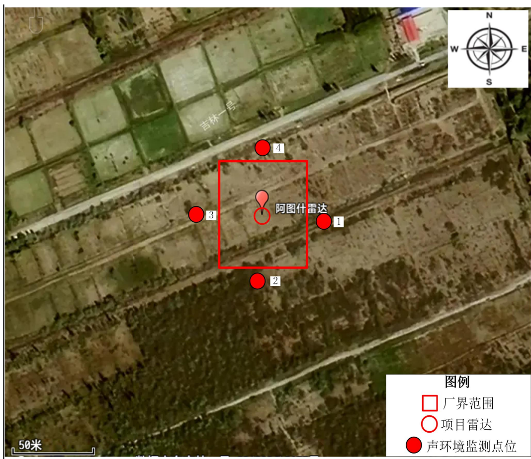
图4-2 噪声监测布点示意图
