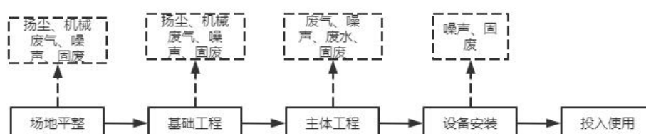
图 3-3 施工期工艺流程及产污节点图
