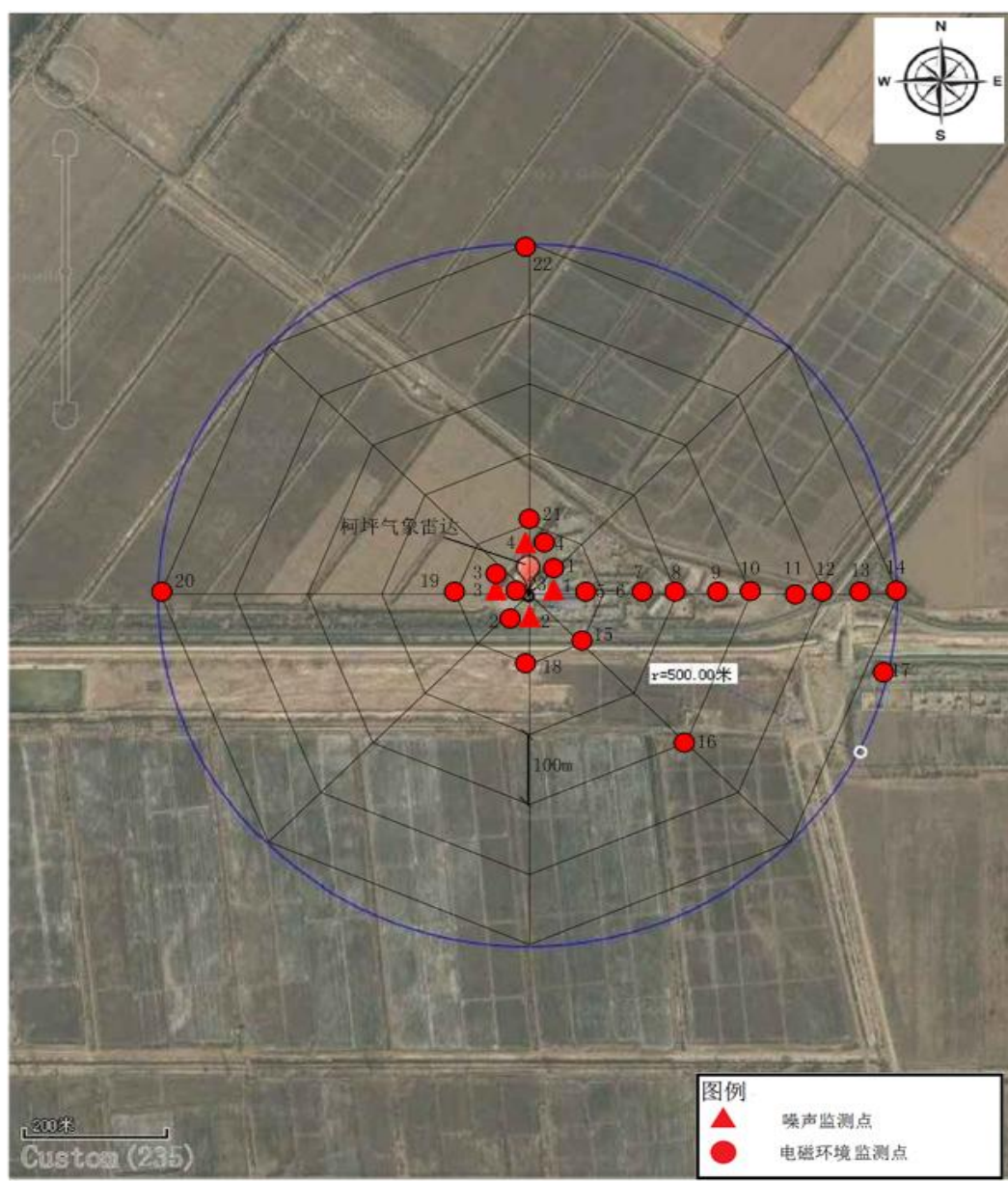
图 6-2 柯坪县雷达站监测点位示意图
