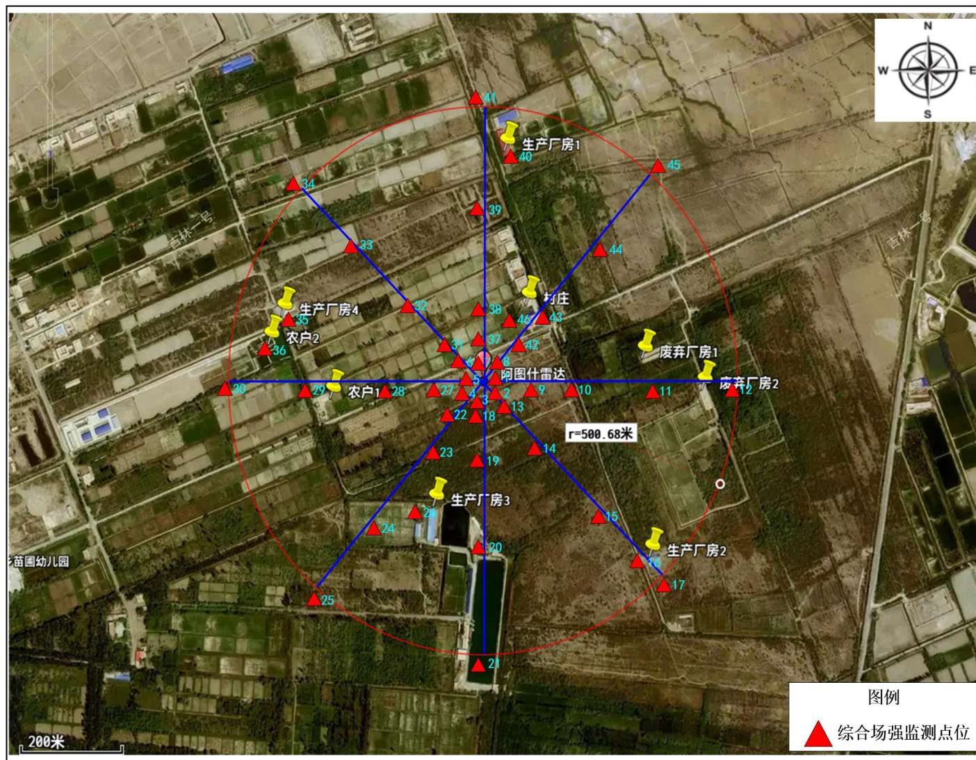
图4-1电磁辐射监测布点示意图
