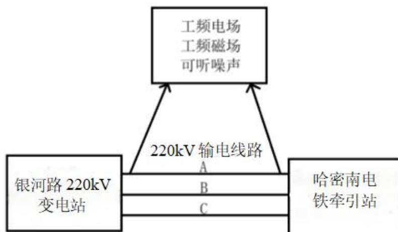
图 3.3-3 220kV 输电线路运行期工艺流程及产污节点图 输电线路施工期和运行期的环境影响要素识别见表 3.3-1。
