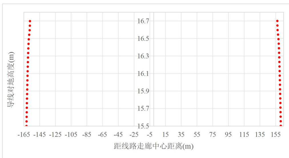
图 6.1-19 4 条单回并行输电线路 10kV/m 等值线图
