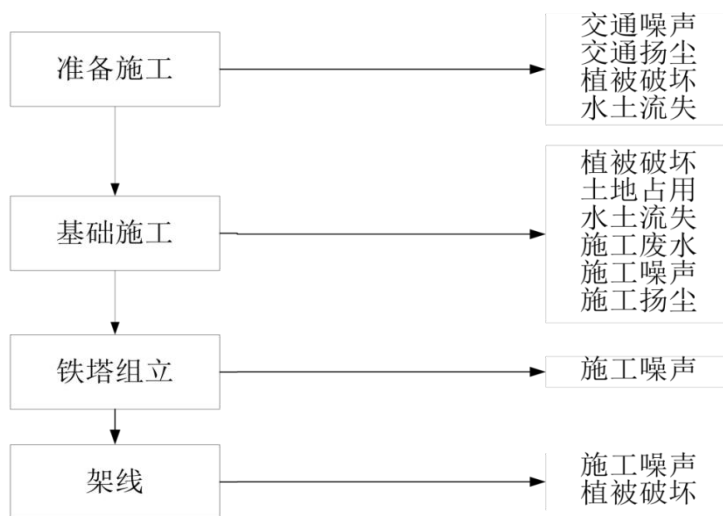
图 3.3-1 输电线路工程施工工艺及产污环节
