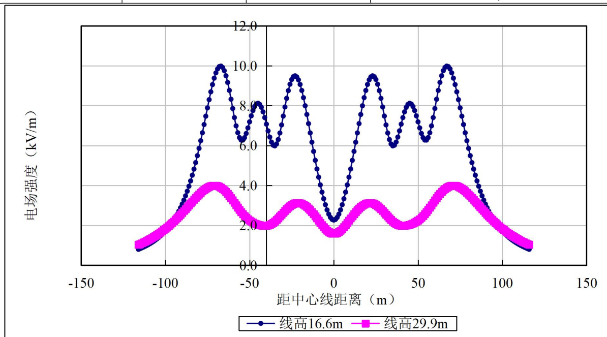
图 6.1-8 750kV 并行单回路输电线路抬升后工频电场强度分布图
