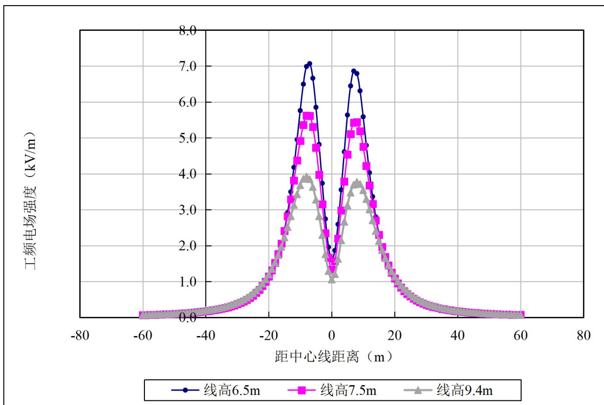
图 6.1-22 220kV 单回路线路工频电场强度预测分布曲线图
