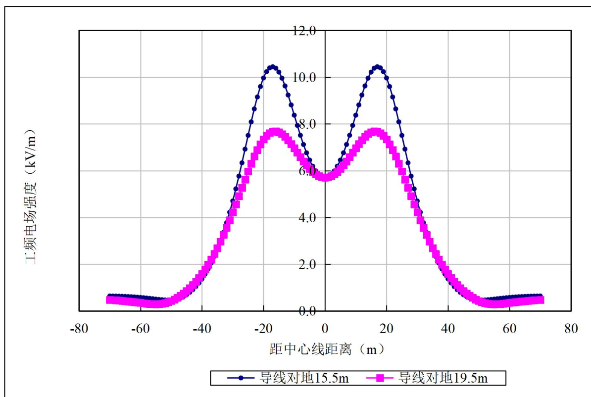
图 6.1-12 750kV 双回路输电线路工频电场强度分布图
