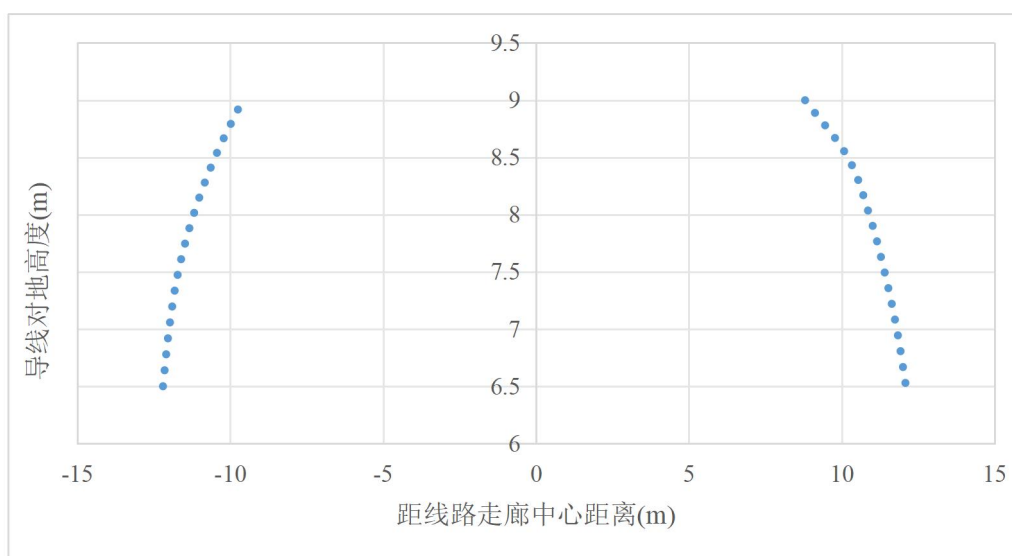
图 6.1-24 220kV 单回路线路 4kV/m 电场强度等值线图
