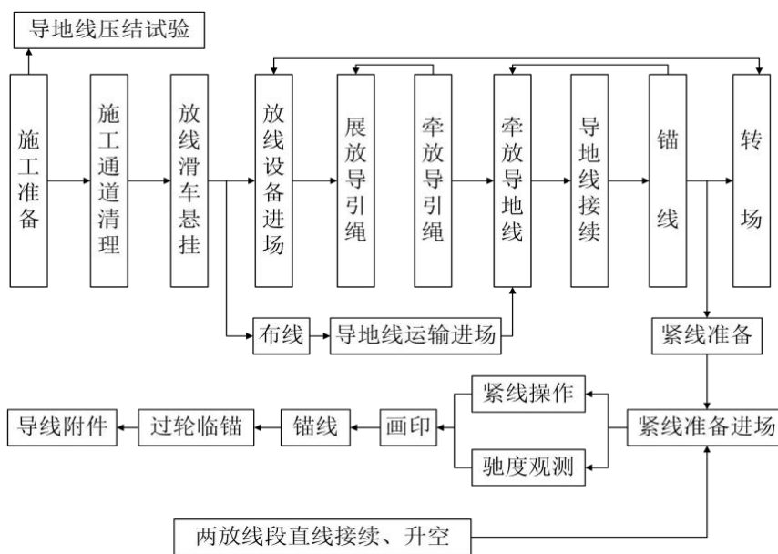
图 3.1-7 架线施工流程图
