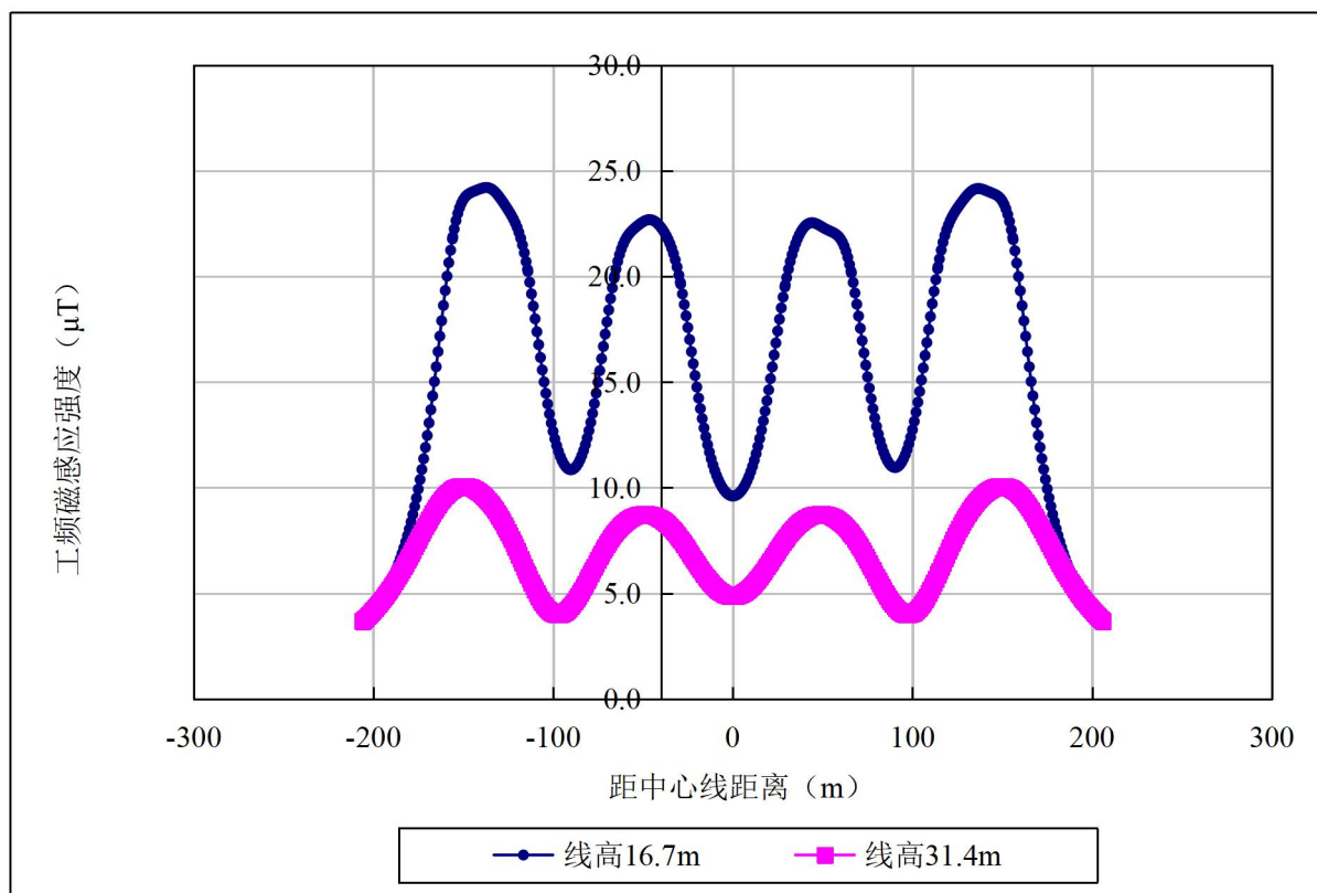
图6.1-21 4条单回并行线路抬升后工频磁感应强度分布图
