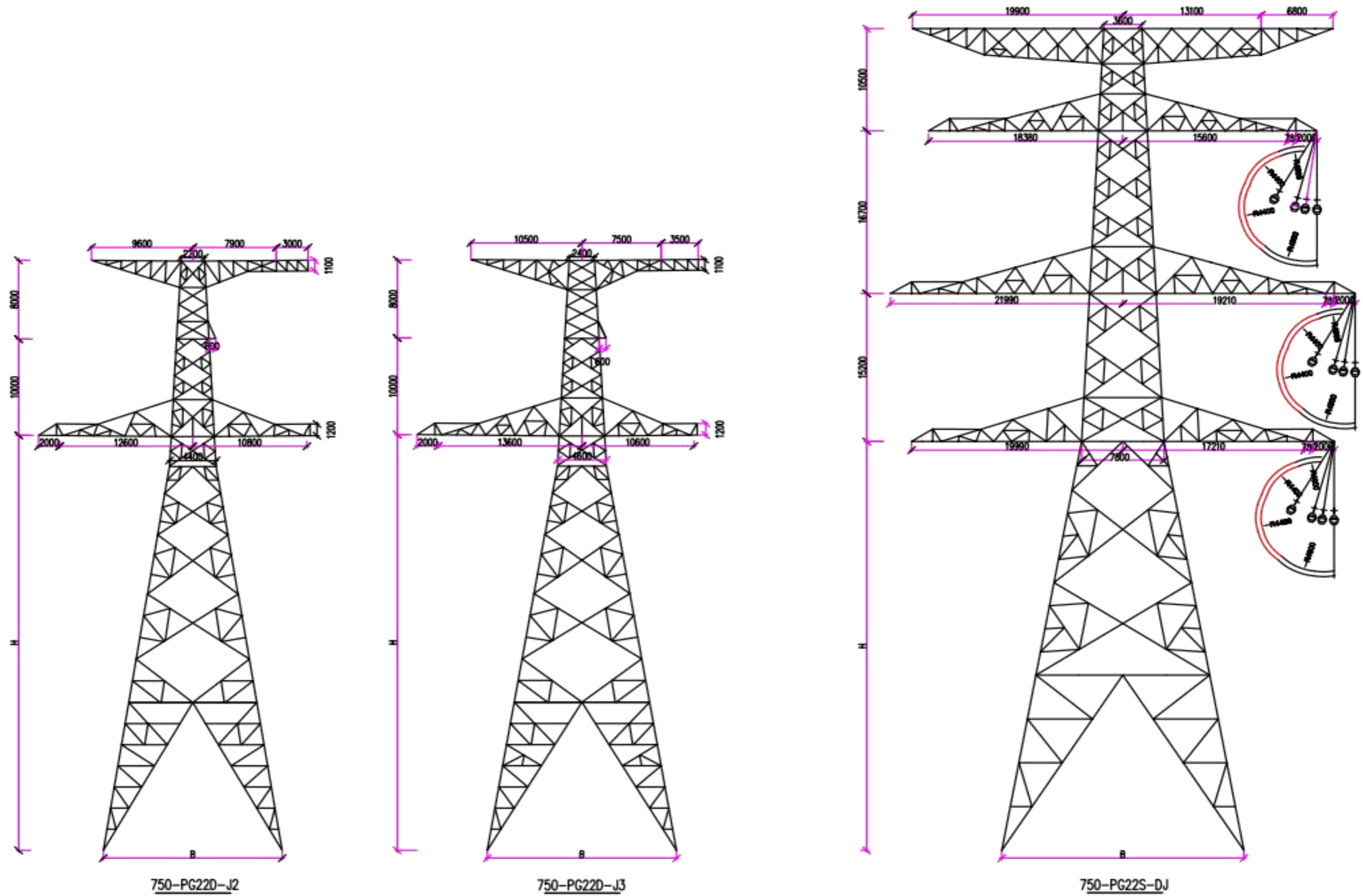
图 3.1-3 750kV 输电线路杆塔一览表
