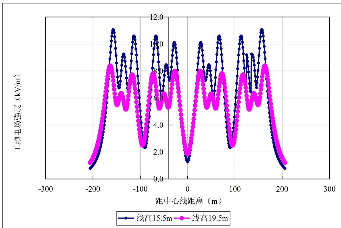
图6.1-17 4条单回并行线路工频电场强度分布图
