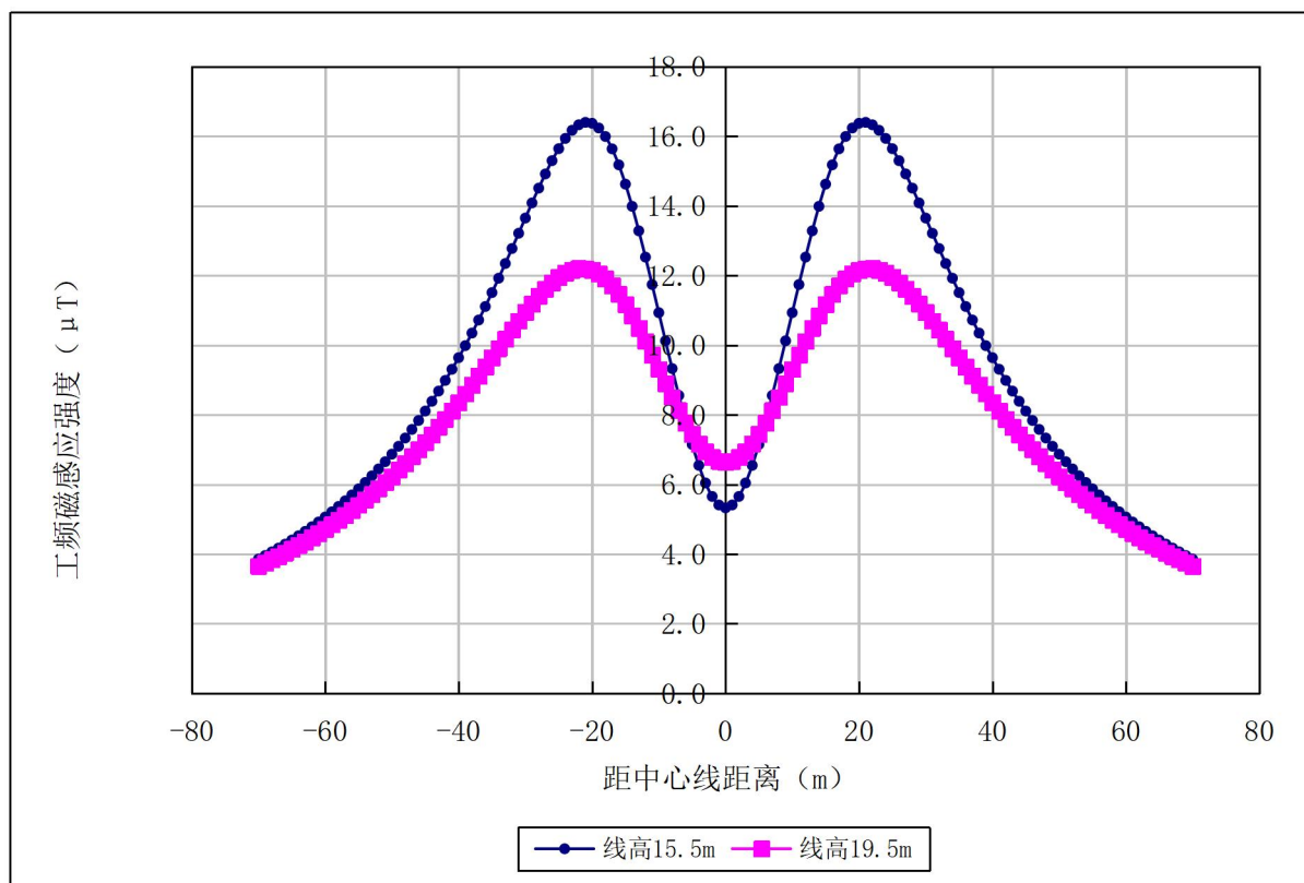
图 6.1-13 750kV 双回路输电线路工频磁感应强度分布图
