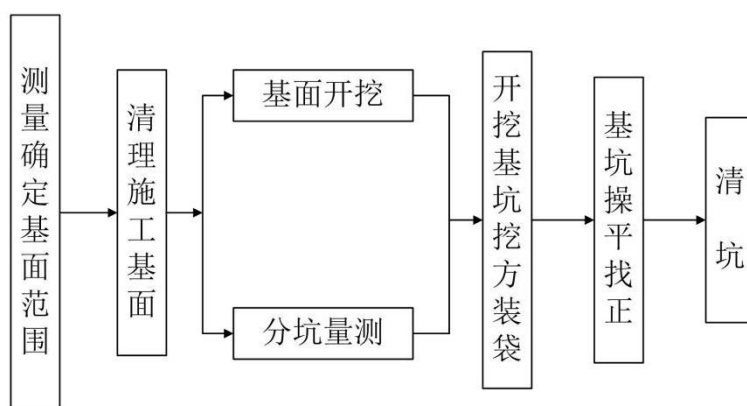
图 3.1-4 基坑开挖施工工艺流程图
