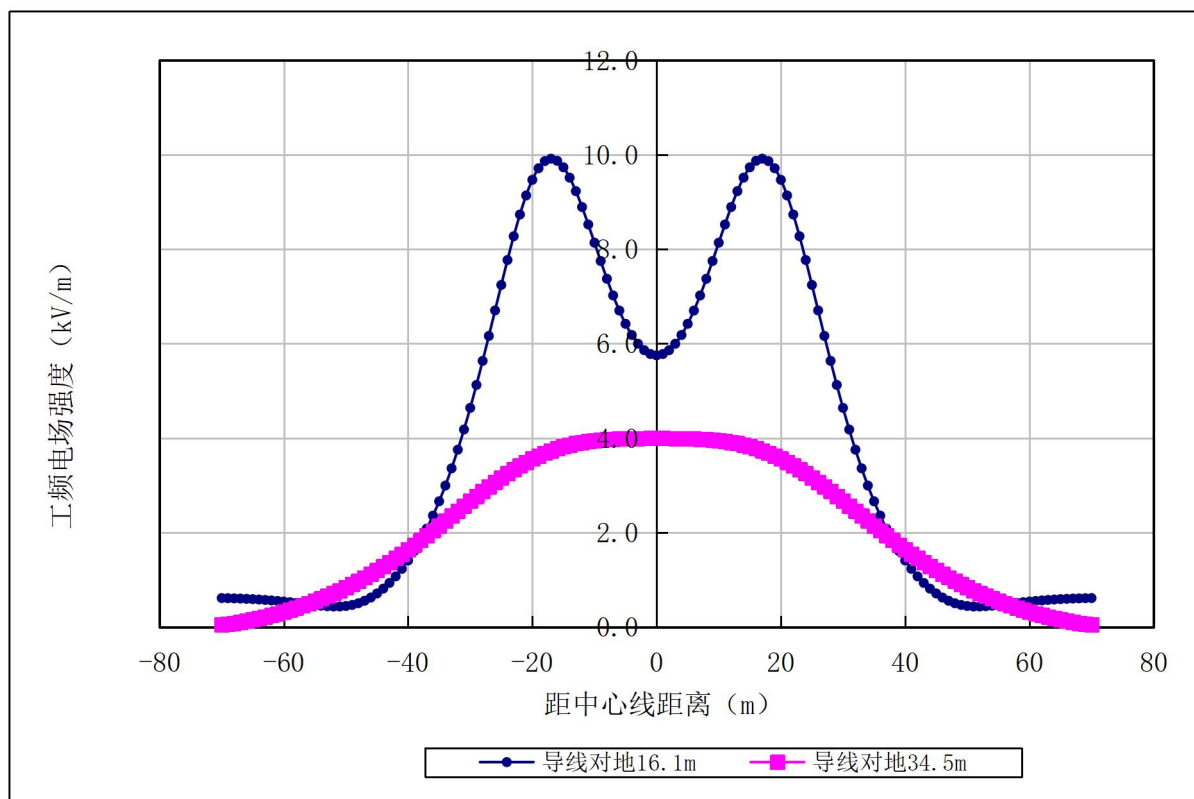
图 6.1-15 750kV 同塔双回路输电线路抬升后工频电场强度分布图
