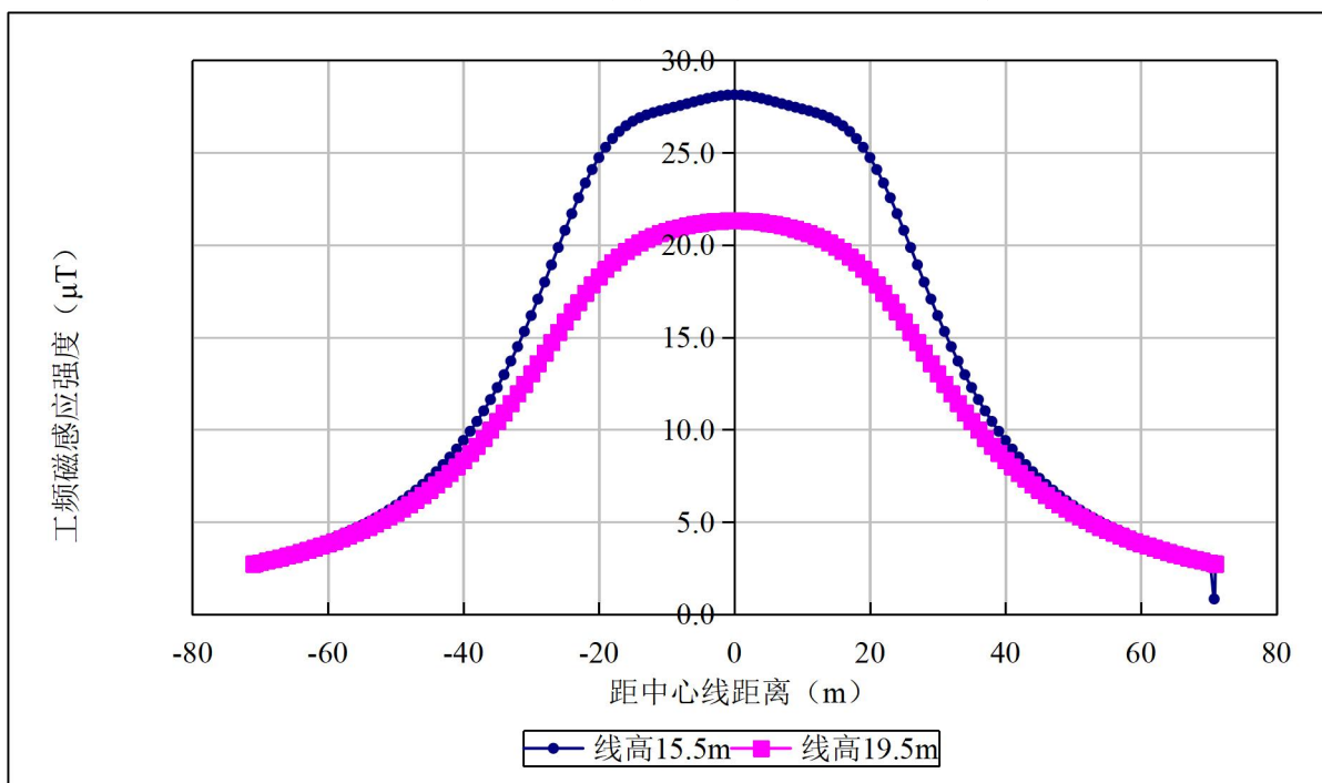
图 6.1-2 750kV 单回路输电线路工频磁感应强度分布图
