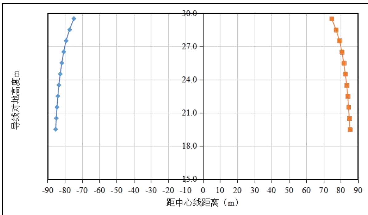
图 6.1-10 750kV 并行单回输电线路 4kV/m 等值线图
