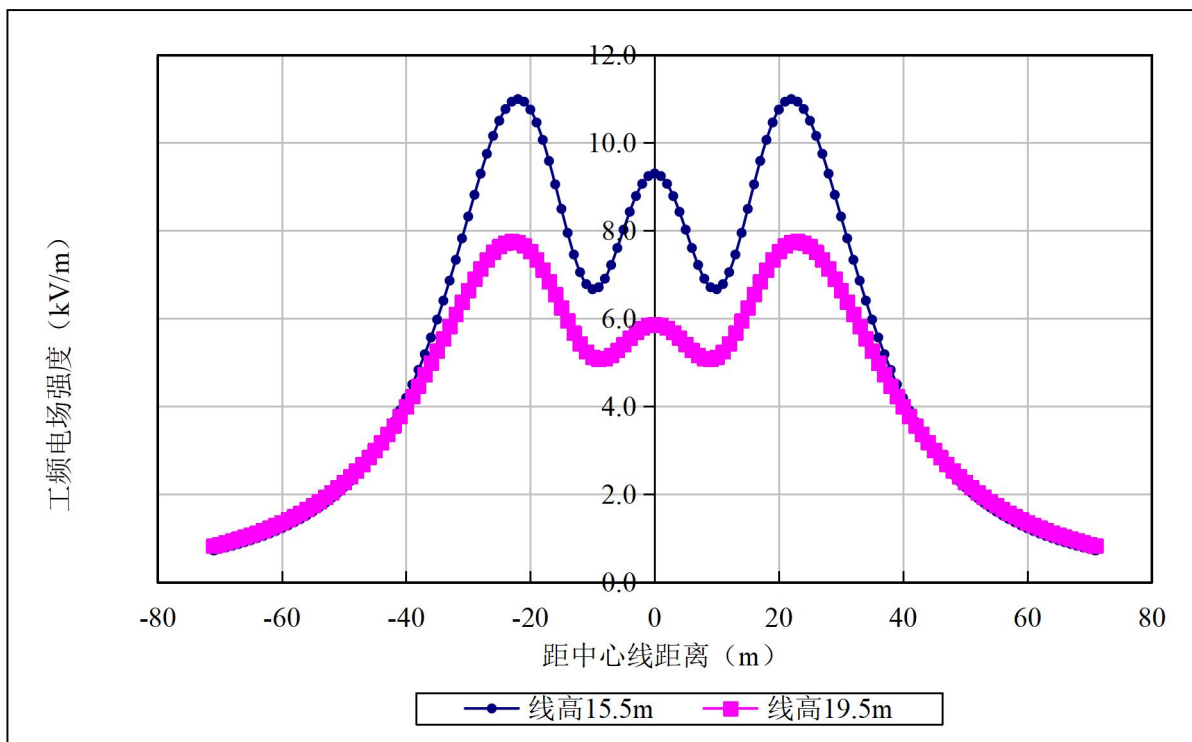
图 6.1-1 750kV 单回路输电线路工频电场强度分布图
