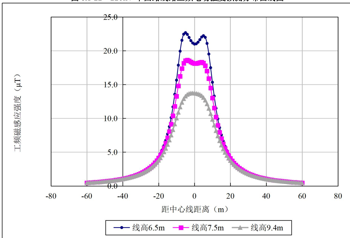
图 6.1-23 220kV 单回路线路工频磁感应强度预测分布曲线图
