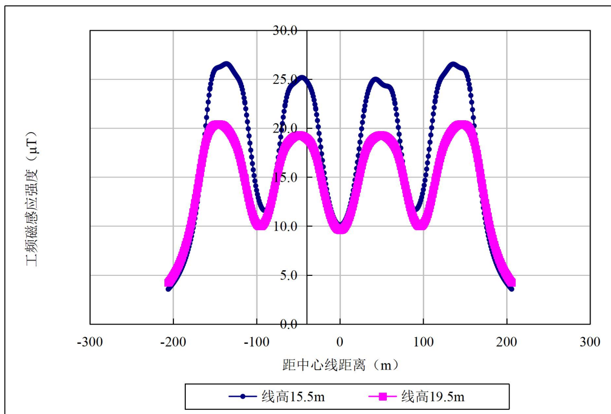
图6.1-18 4条单回并行线路工频磁感应强度分布图（非居民区）
