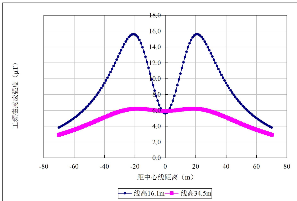
图 6.1-16 750kV 同塔双回路输电线路抬升后工频磁感应强度分布图
