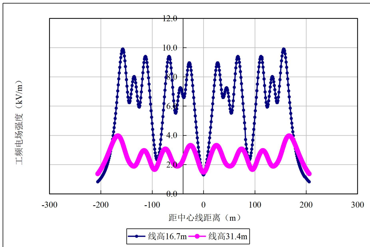
图6.1-20 4条单回并行线路抬升后工频电场强度分布图
