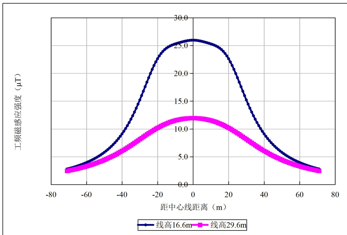
图 6.1-4 750kV 单回路输电线路抬升后工频磁感应强度分布图
