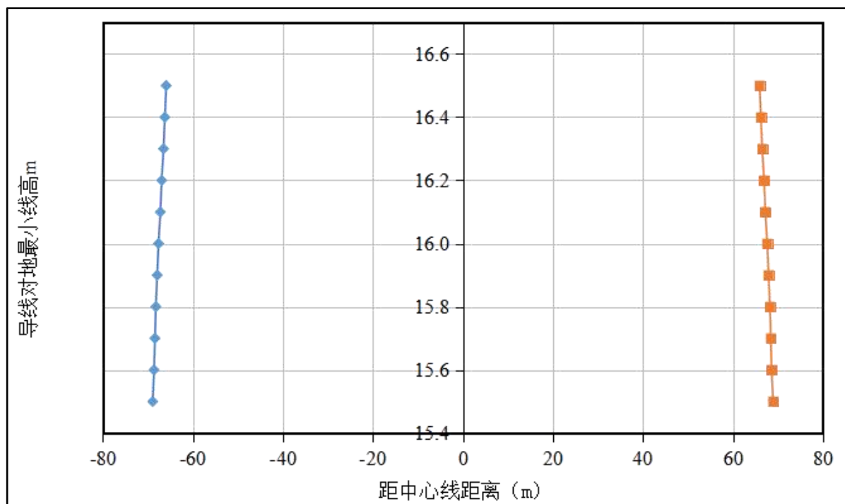
图 6.1-11 750kV 并行单回输电线路 10kV/m 等值线图
