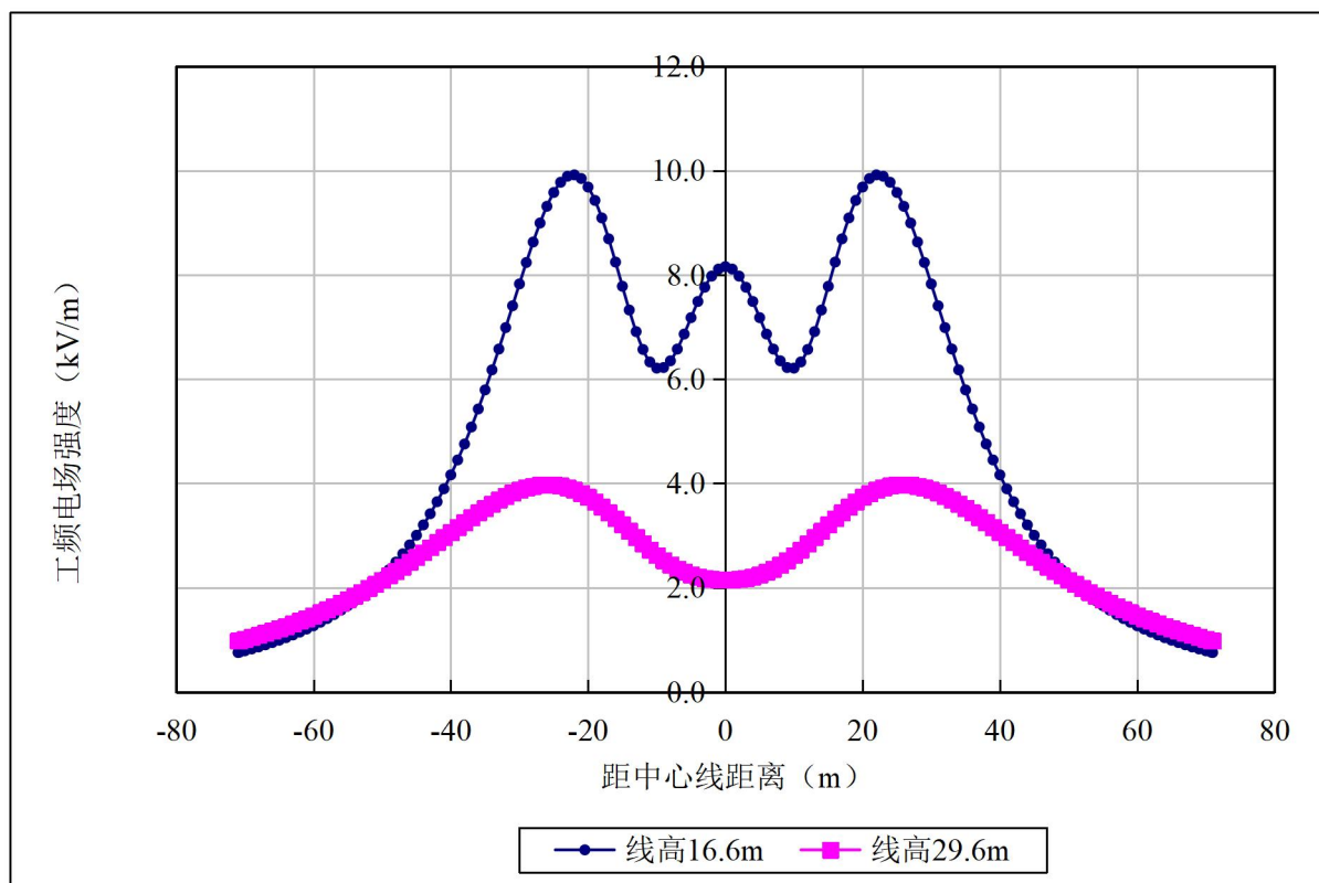
图 6.1-3 750kV 单回路输电线路抬升后工频电场强度分布图
