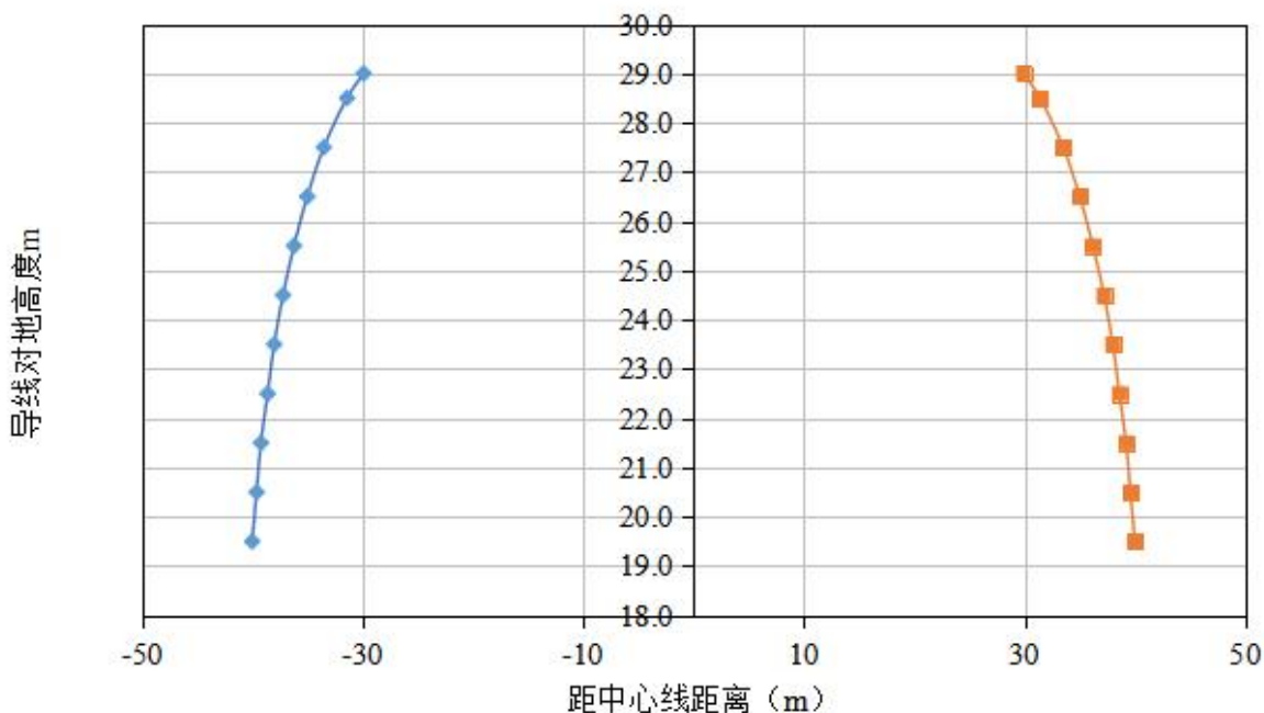
图 6.1-5 750kV 单回路输电线路 4kV/m 等值线图
