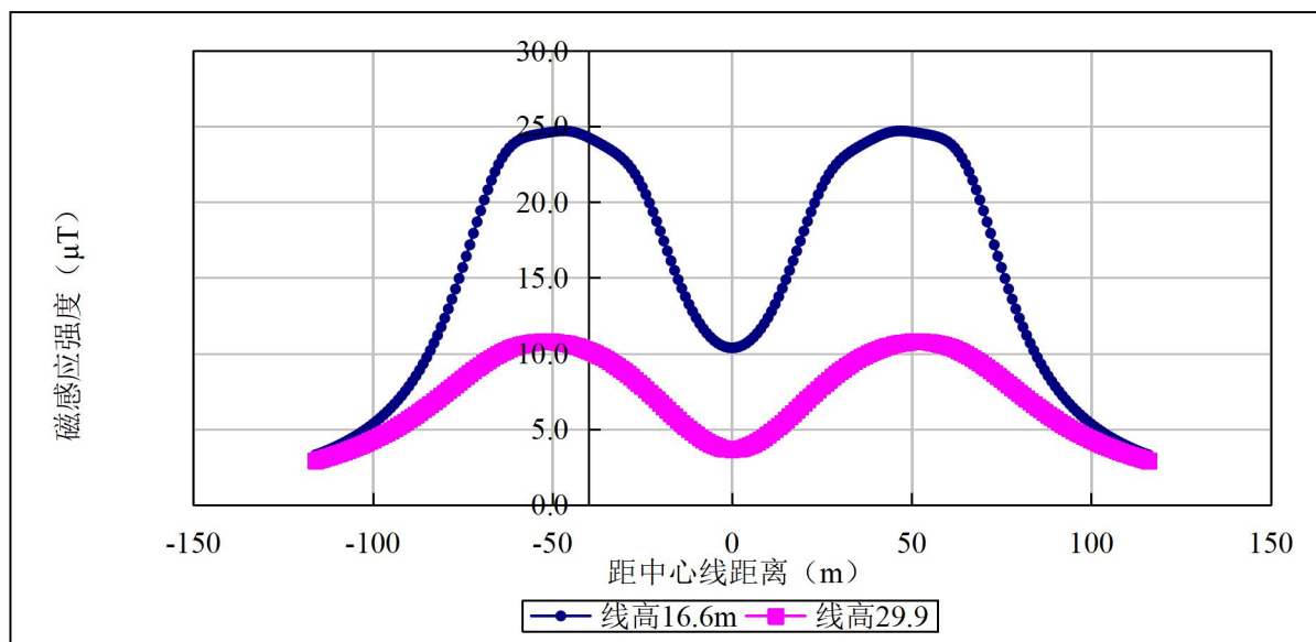
图 6.1-9 750kV 并行单回输电线路抬升后工频磁感应强度分布图
