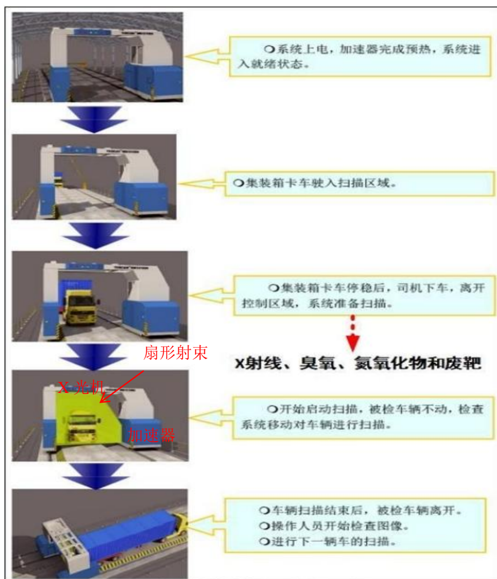
图 9-7 同类型集装箱/车辆检查系统精细检查模式下的工作流程及产污示意图
