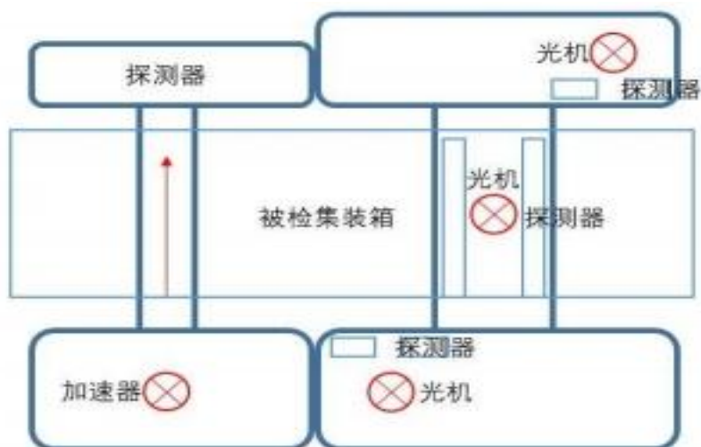
图 9-4 设备构成示意图
