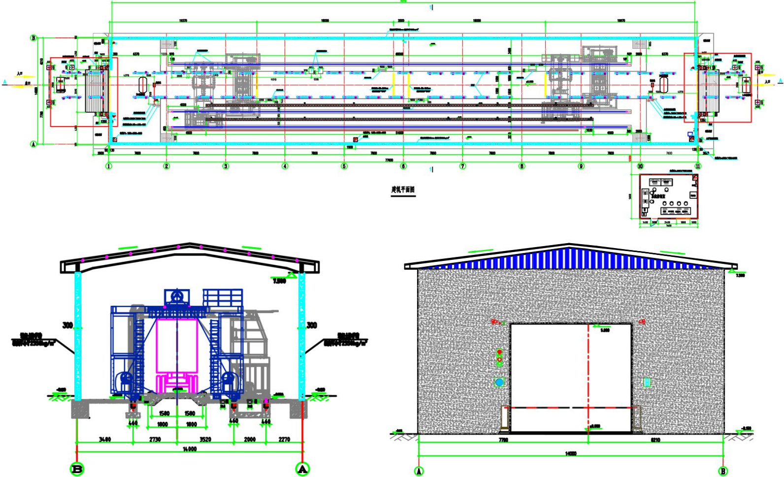
附图 4 扫描大厅平面图
