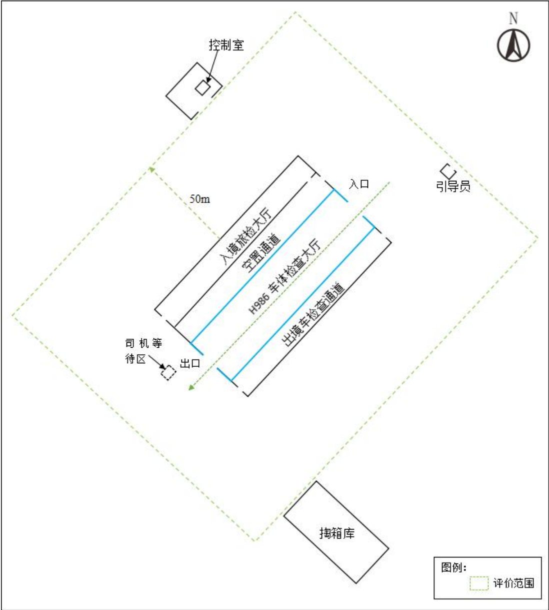
附图 3 建设项目平面布局图
