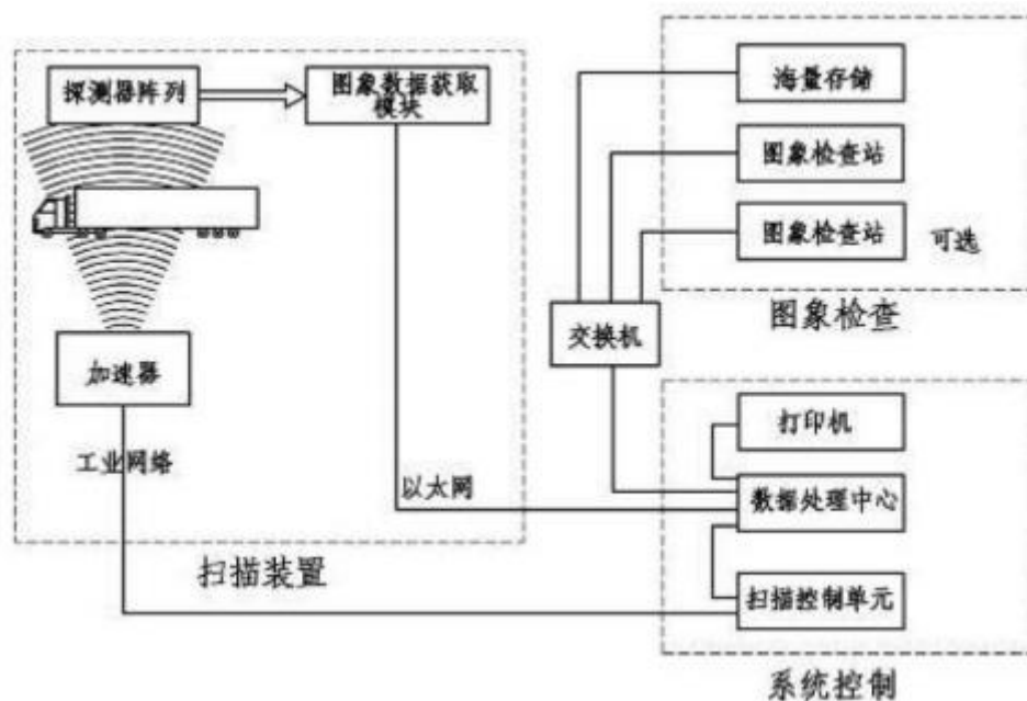
图 9-5 X 射线成像分系统示意图
