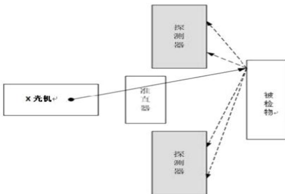
图 9-3 MB1215DE (BX) 系统 X 射线背散射成像系统示意图
