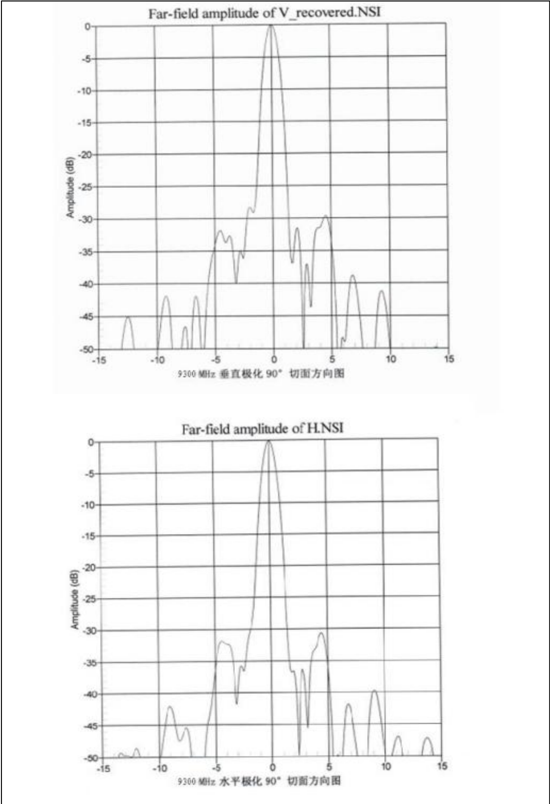
附图8 天气雷达天线方向图
