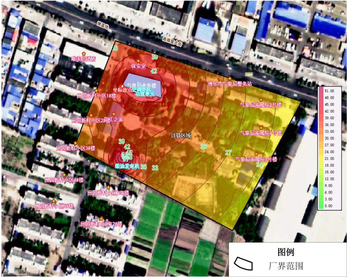
图6-5 噪声贡献值等值线图
