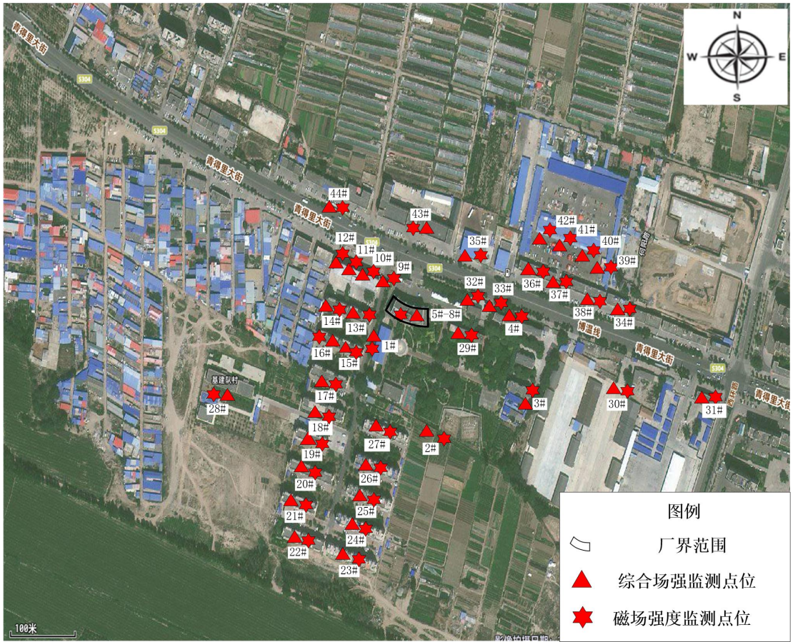
图4-1电磁辐射监测布点示意图
