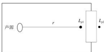
图 6-4 室内声源等效为室外声源图例
