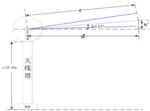
图6-1 近场区天线前方限高计算示意图
