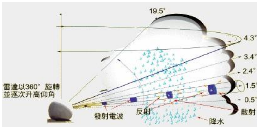
图 3-5 X 波段气象雷达系统工作原理图
