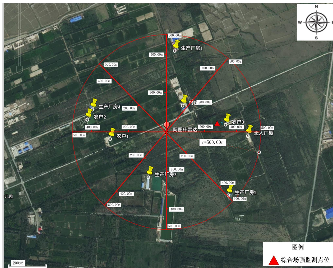
图4-1电磁辐射监测布点示意图（2）
