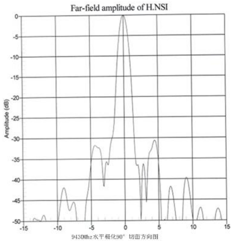
附图 8 天线水平、垂直方向图
