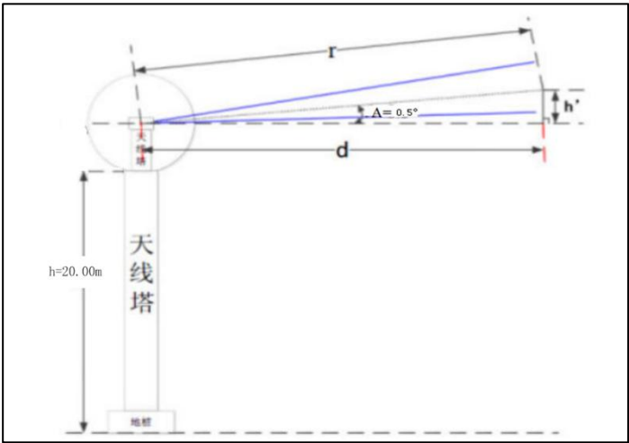
图6-1 天线前方限高计算示意图
