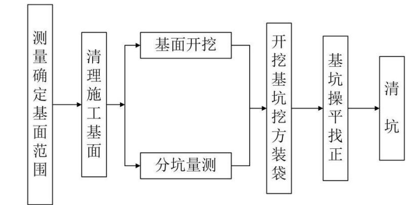
图 3.1-9 基坑开挖施工工艺流程图
