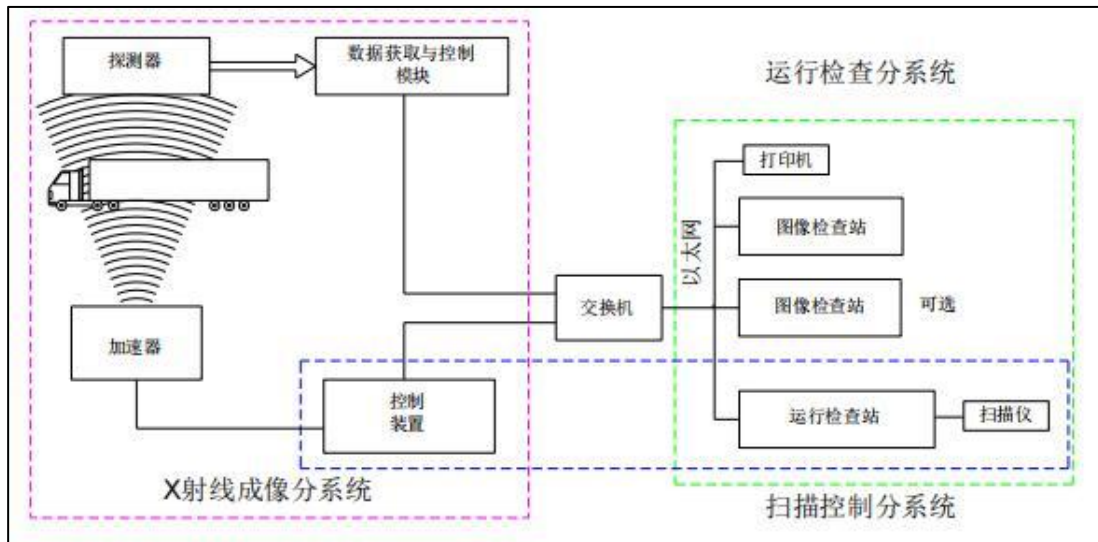
图9-1 检查系统的构成及逻辑机构
