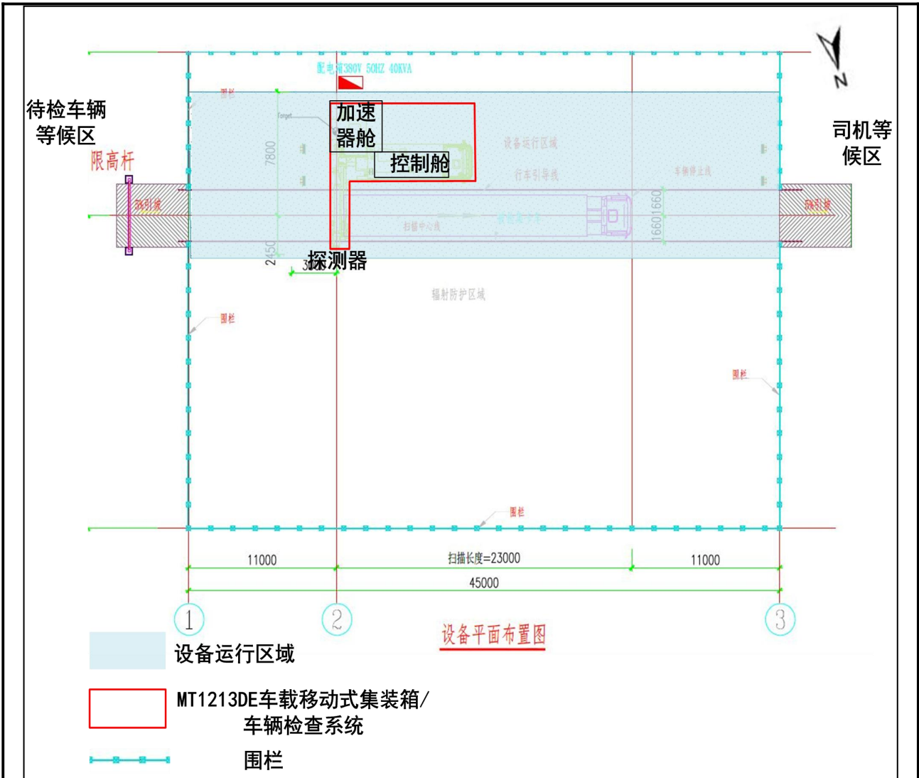
图10-2 车辆检查装置平面布置示意图
