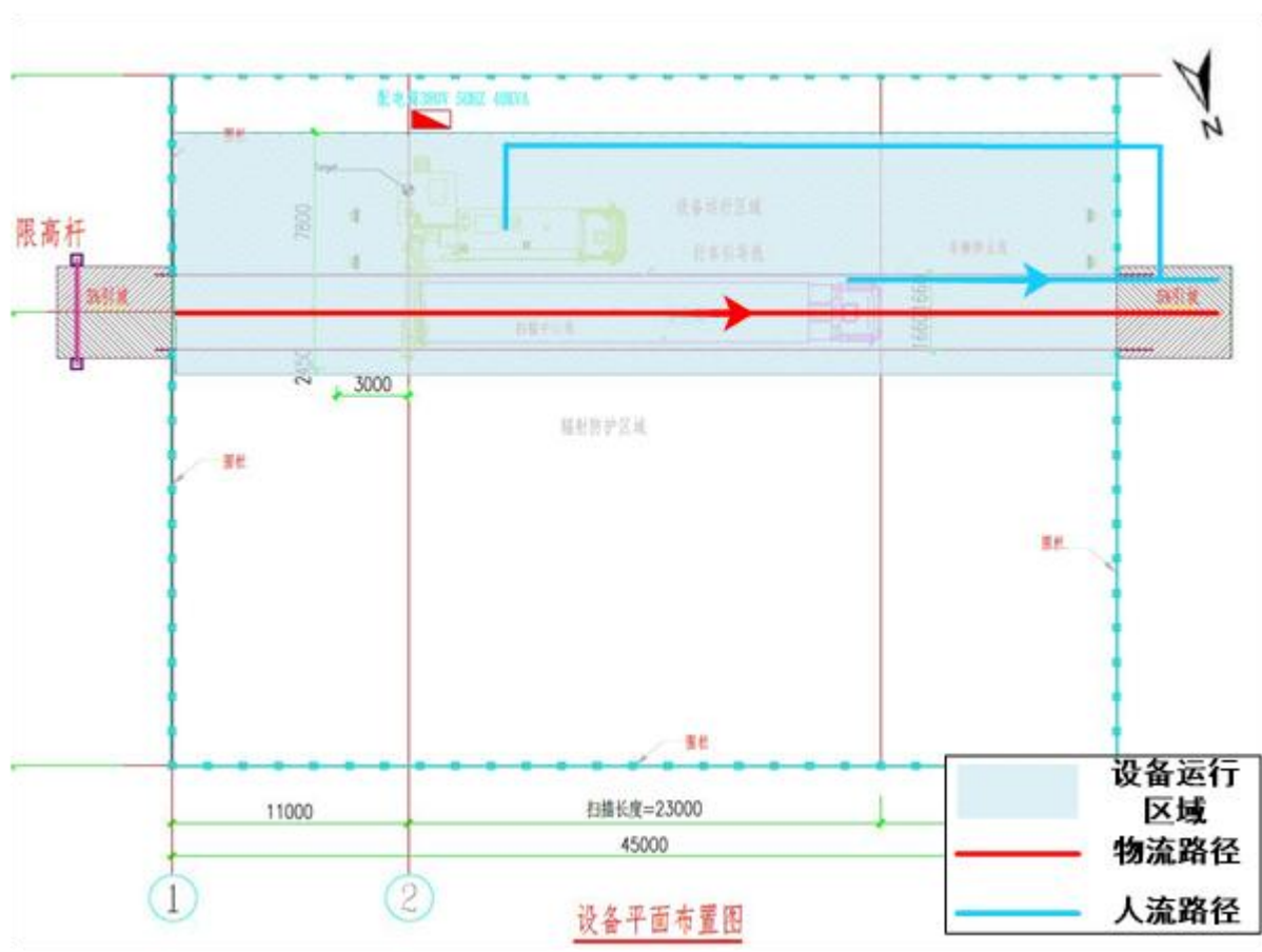
图9-5 MT1213DE安全检查系统的人流、物流路径图
