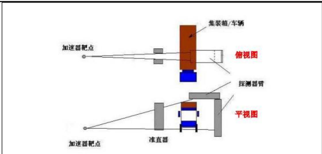
图9-2 MT1213DE检查系统X射线成像分系统示意图
