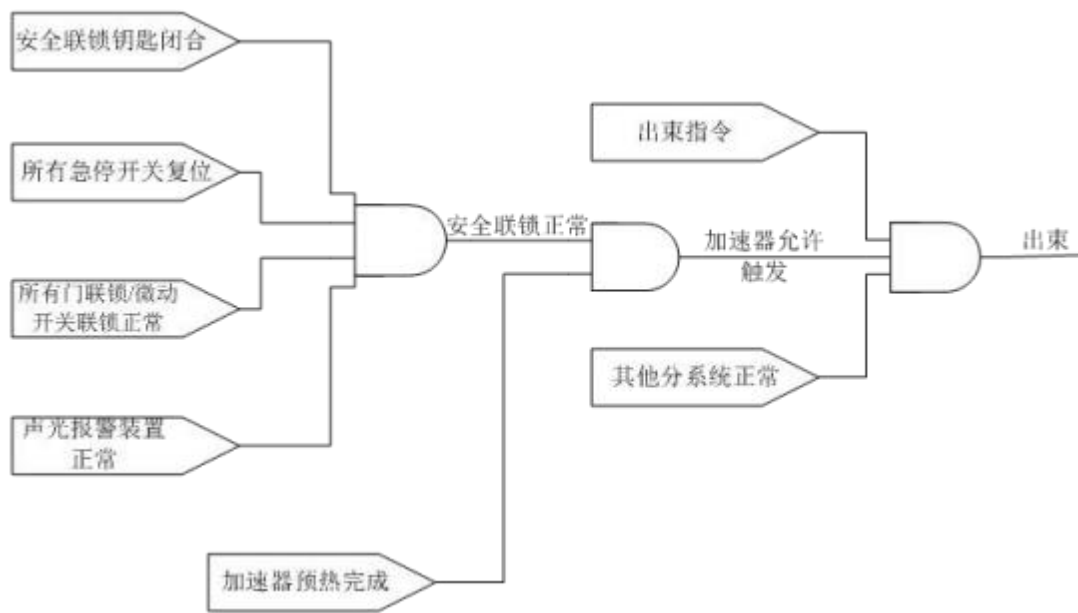
图10-4 MT1213DE 型集装箱/车辆检查系统安全联锁逻辑图
