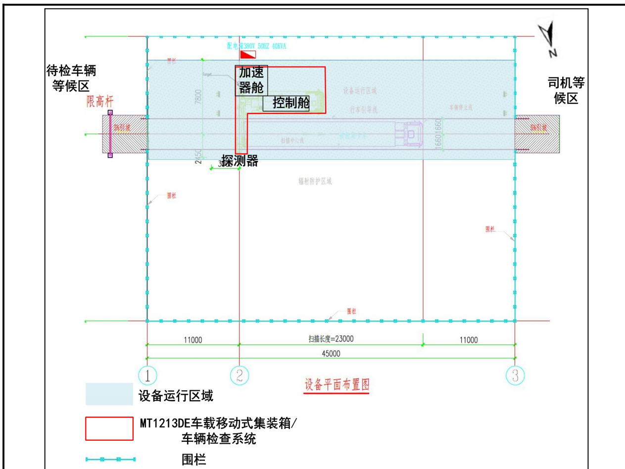
图1-4 MT1213DE车载移动式集装箱/车辆检查系统平面设计图
