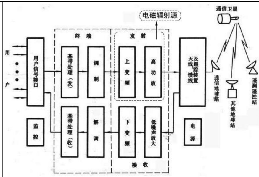
图 2-3 卫星地面站发送传输信号流程示意图
