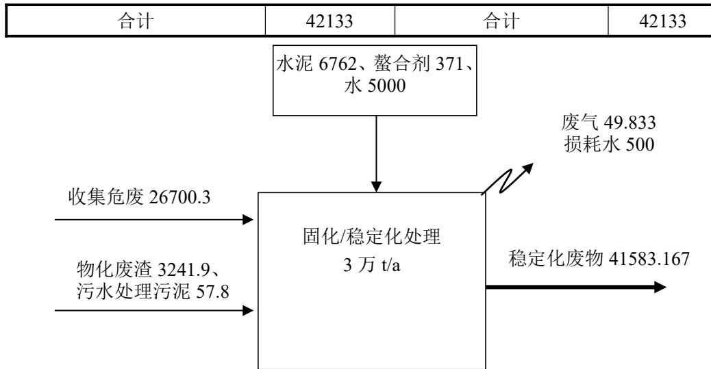
图 4.6-2 稳固化车间物料平衡 单位：t/a
