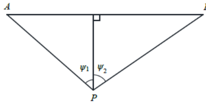
图 5.5-1 有限路段的修正函数，A~B 为路段，P 为预测点
