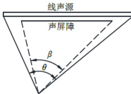
图 5.5-5 受声点与线声源两端连接线的夹角（遮蔽角）
