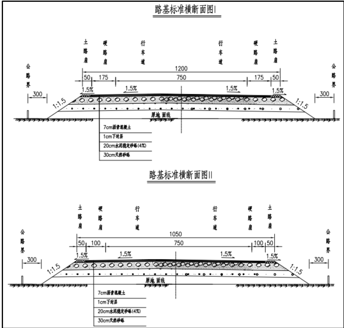
图3.1-1 路基标准横断面图
