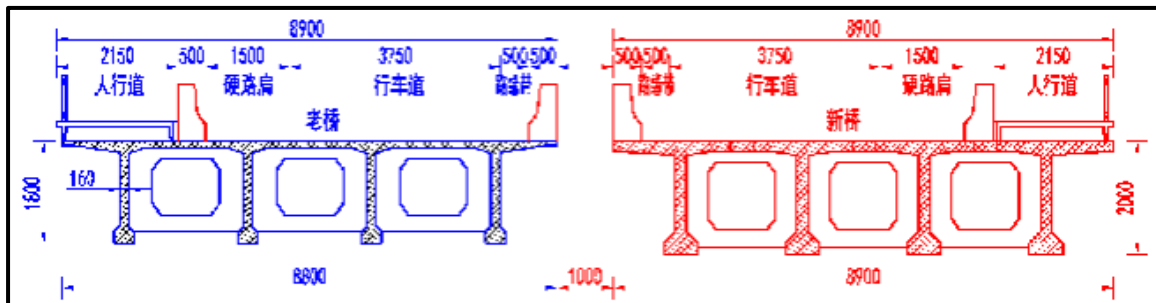
图 3.1-5 方案二横断面布置图
