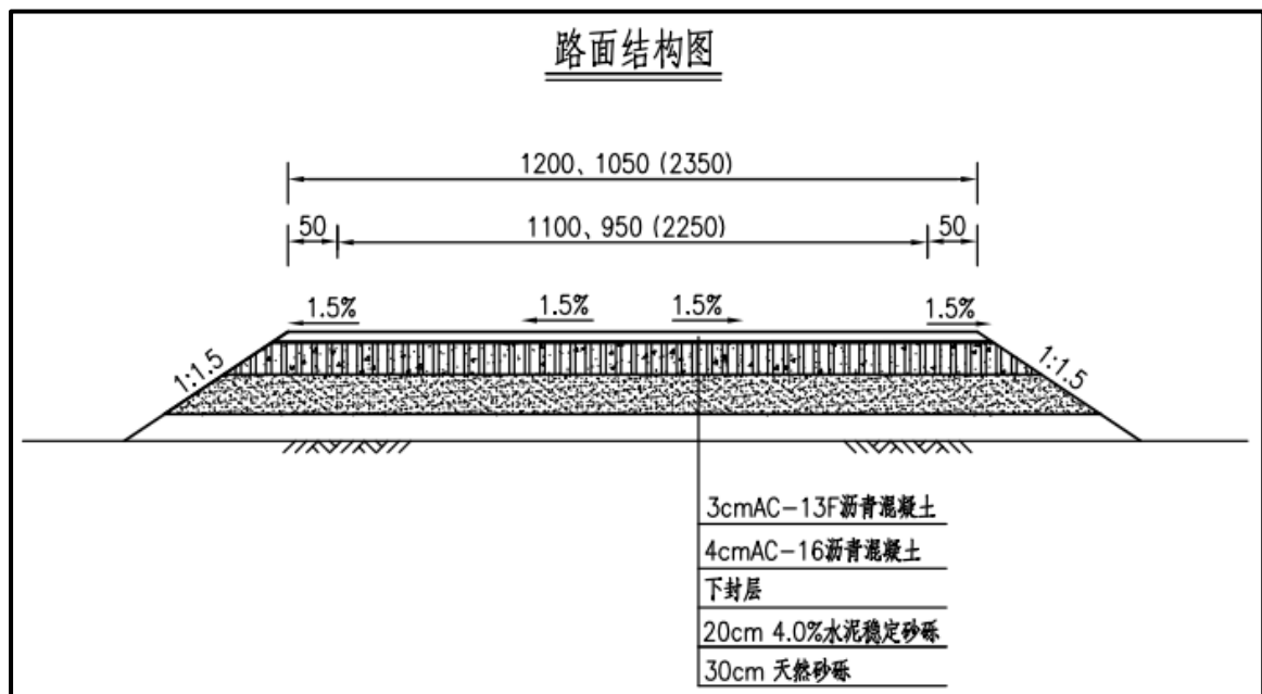
图3.1-2 路面结构图
