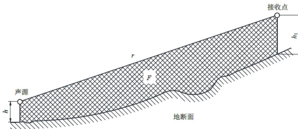
图 5.5-6 估计平均高度 h_m 的方法
