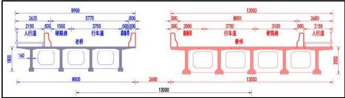
图 3.1-6 方案三横断面布置图
