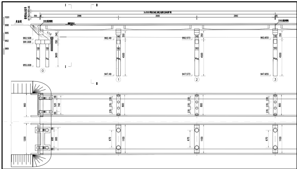
图3.1-3 大桥桥型结构图
