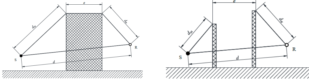
图 5.5-4 利用建筑物、土堤作为厚屏障
