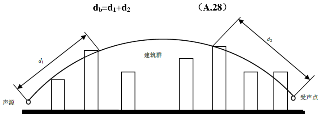
图 5.5-8 建筑群中声传播路径
