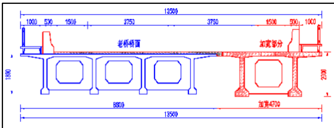
图 3.1-4 方案一横断面布置图
