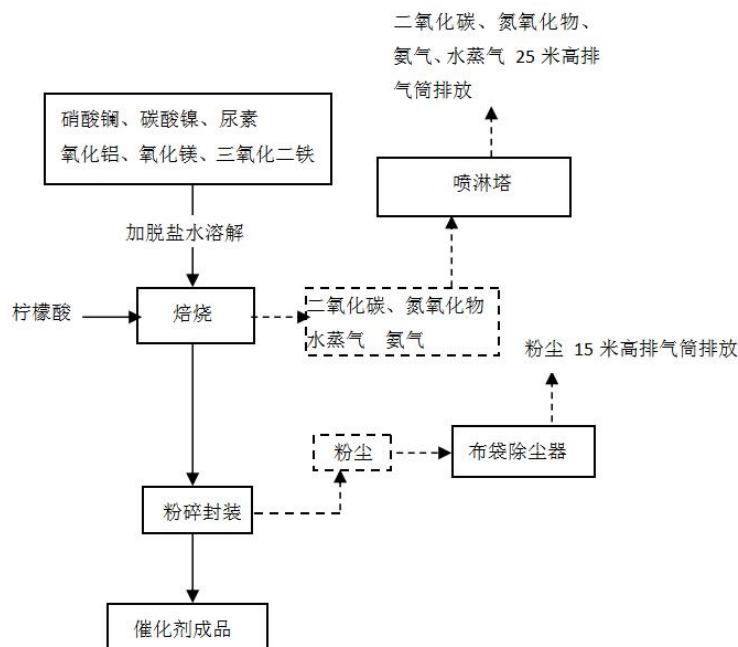
图 3.1-1 催化剂生产工艺及产污流程图
