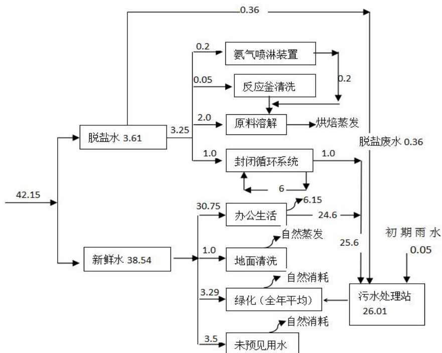
图3.1-4 拟建项目水平衡 单位： m^3/d
