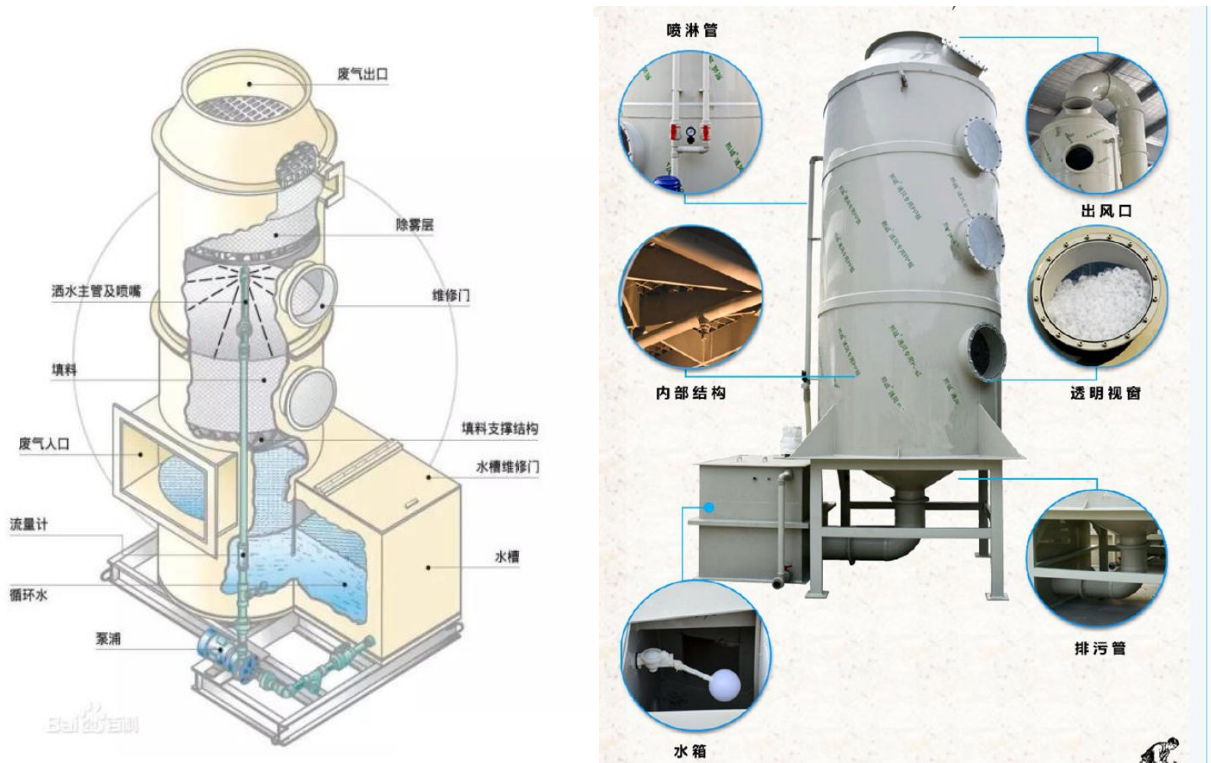
图 7.2-1 两级喷淋塔剖面图和外观图
