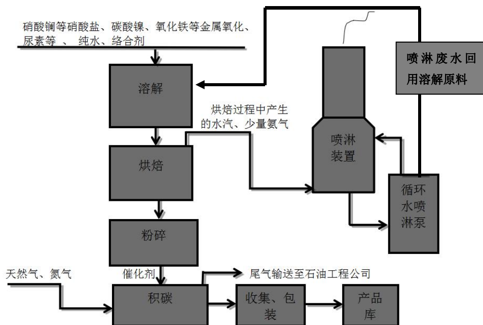
图 3.1-2 总体工艺流程图
