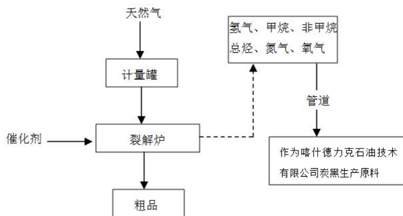
图3.1-3 裂解工序物料转化示意图
