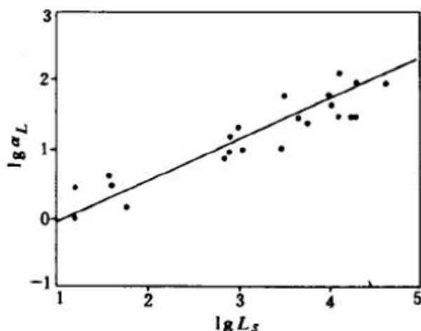
图5.2-1 孔隙介质数值模型的 \lg \alpha L - \lg L_s
