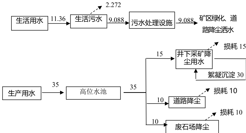
图 2.2-3 本项目水平衡图 (单位: \text{m}^3/\text{d} )
