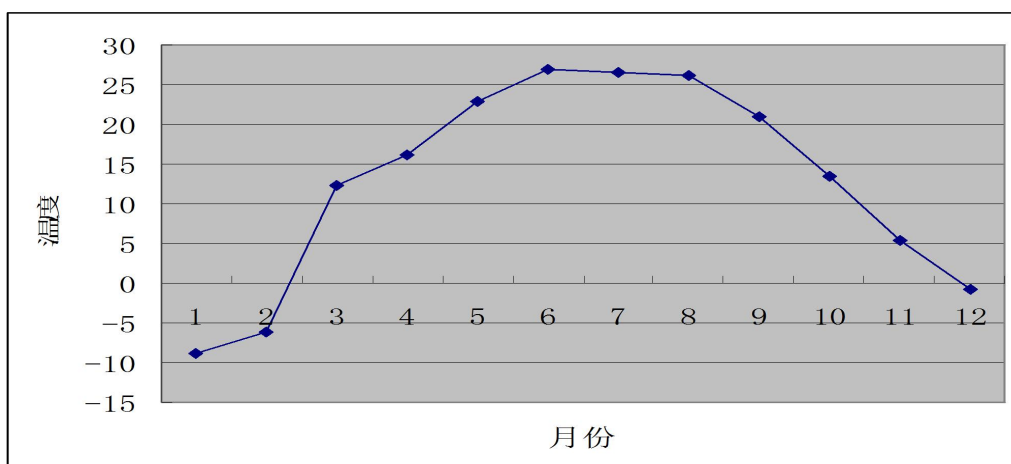
图 4.2-4 平均温度月变化曲线图
