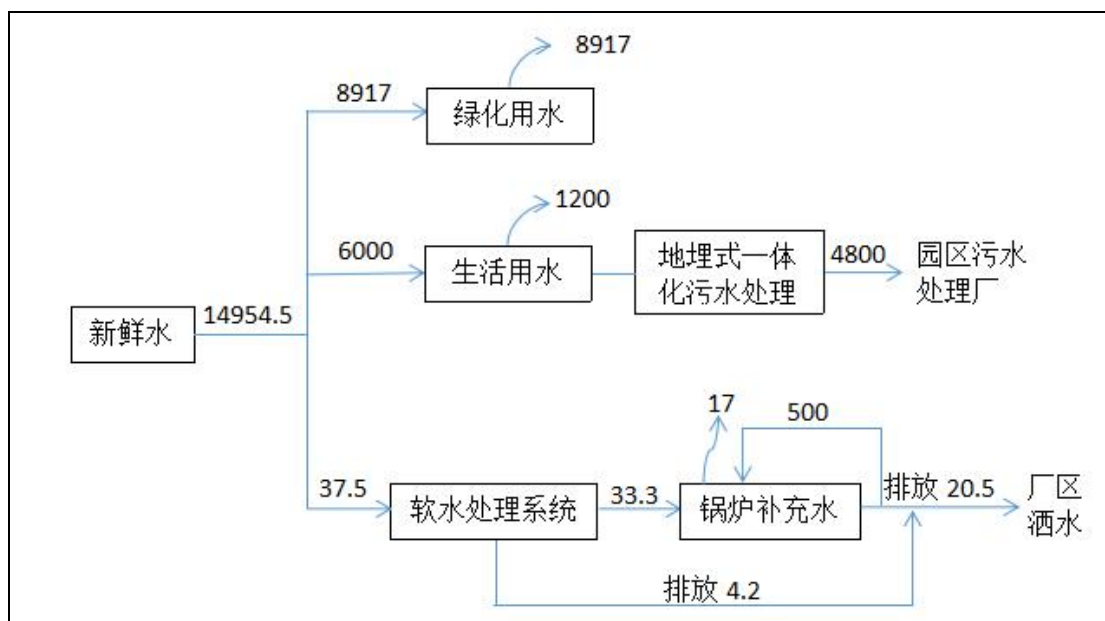
图 2.3-3 项目水平衡图（冬季，150d） 单位：m 3 /a
