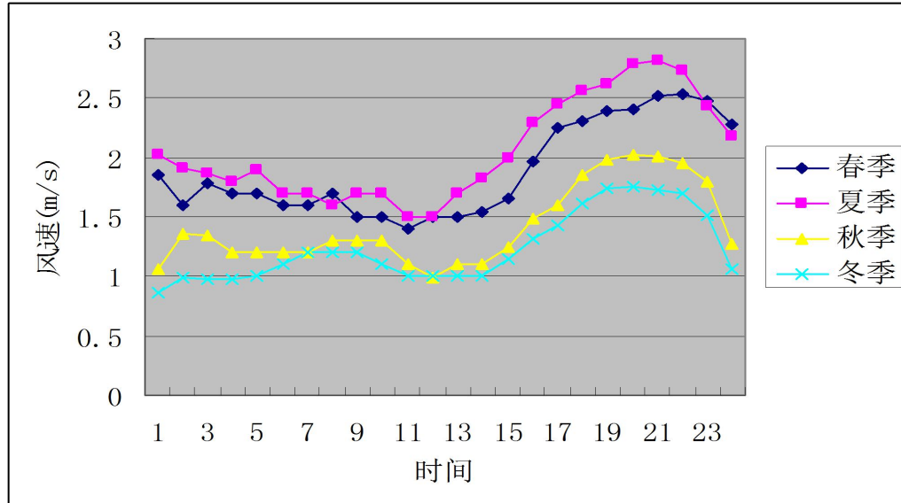
图 4.2-1 平均风速月变化曲线图
