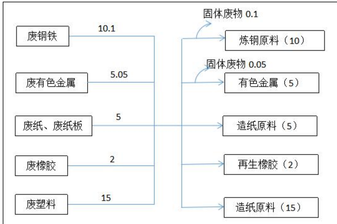
图 2.2-1 项目物料平衡图（单位：万 t/a）
