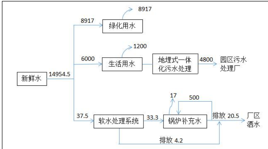
图 2.3-3 项目水平衡图（冬季，150d） 单位：m³/a
