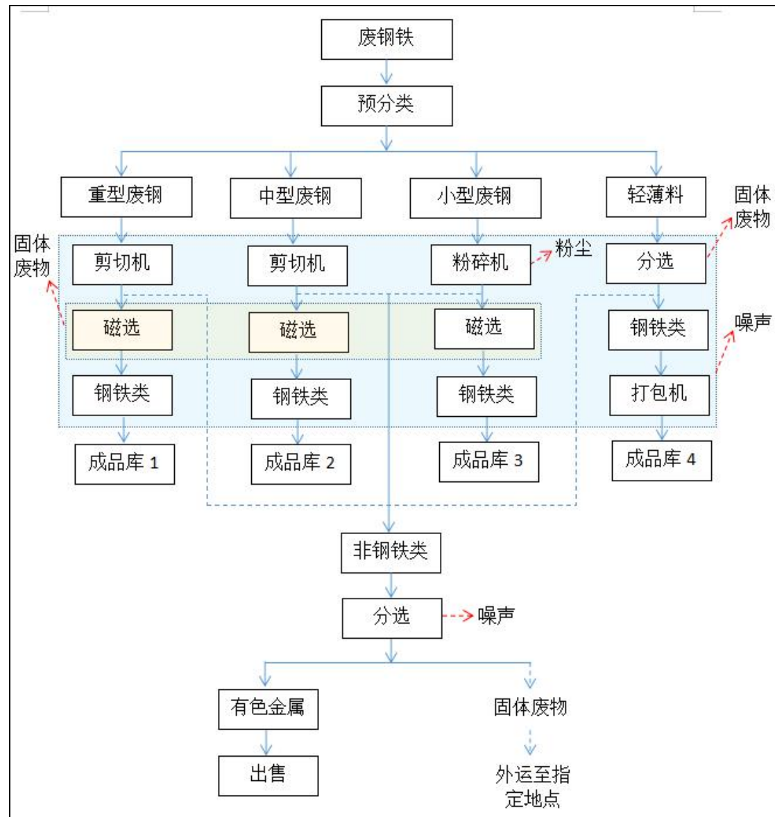
图 2.3-1 废钢铁、废有色金属回收利用工艺流程图
