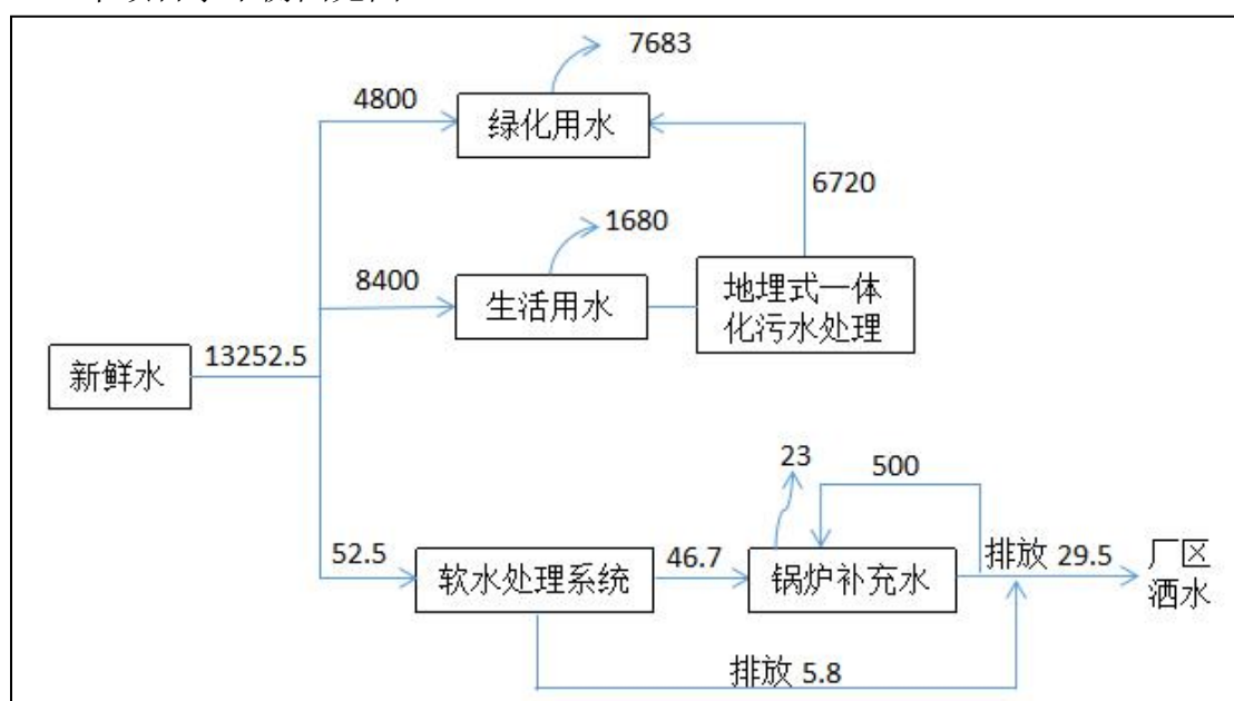
图 2.3-3 项目水平衡图（夏季，210d） 单位：m 3 /a
