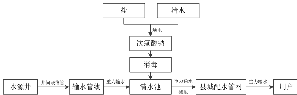
图 3.4-4 运营期生产工艺流程及产污环节图
