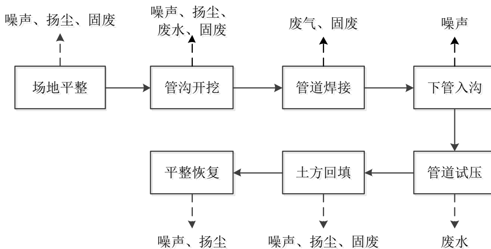
框图 3.4-2 管线施工工序及产污环节图
