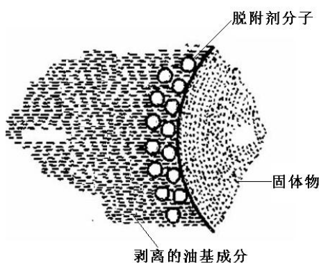
图3.3-2 脱附剂作用机理示意图
