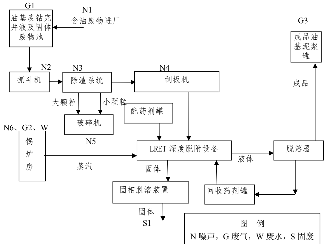
图 3.3-3 LRET 工艺生产流程图
