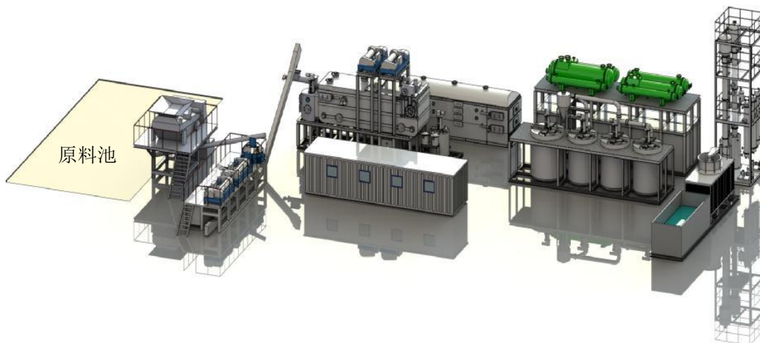
图 3.3-1 LRET 工艺成套装置效果图
