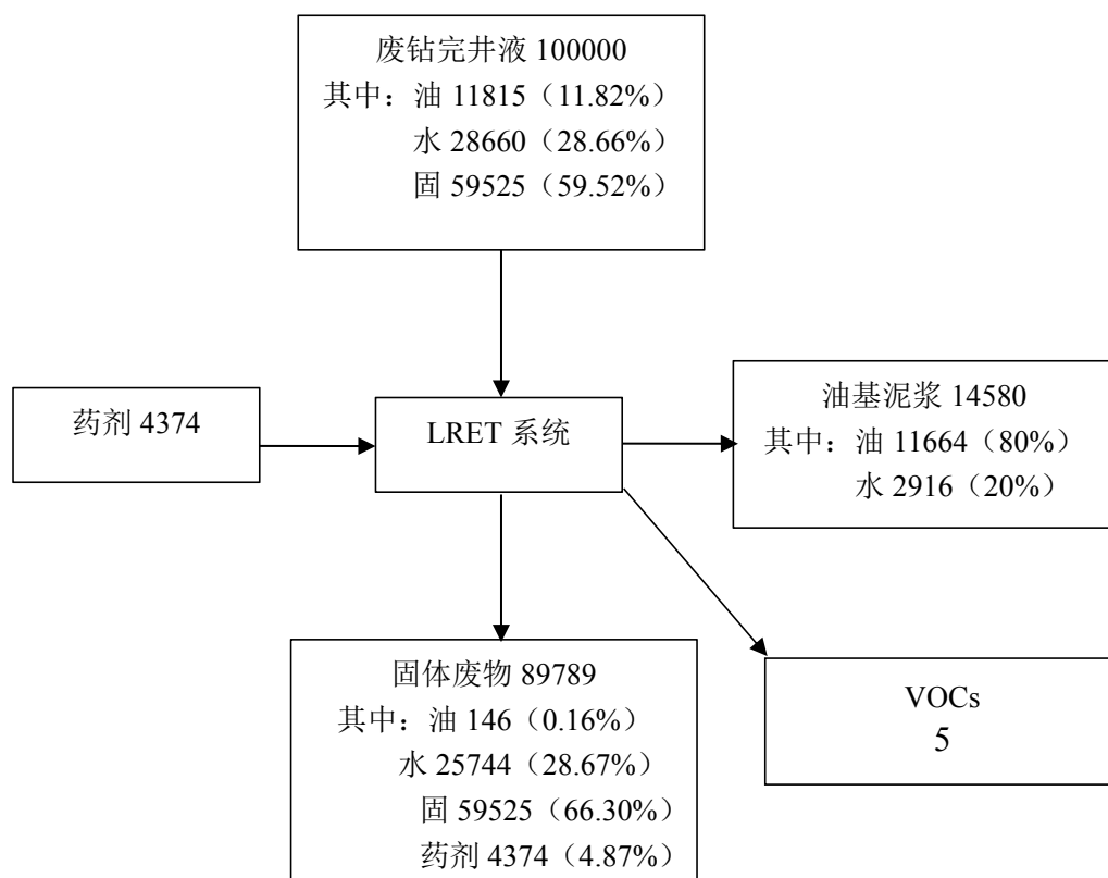
图 3.3-4 LRET 技术工艺流程图 (单位: t/a)
