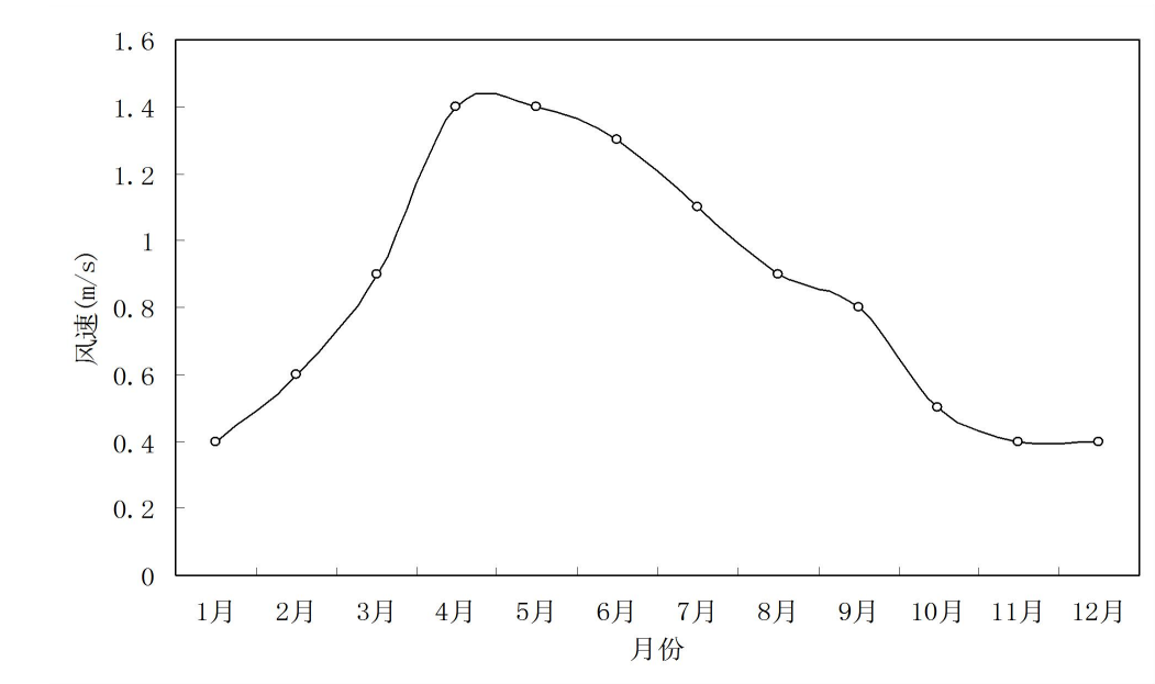
图 5.2-3 多年平均风速的月变化
