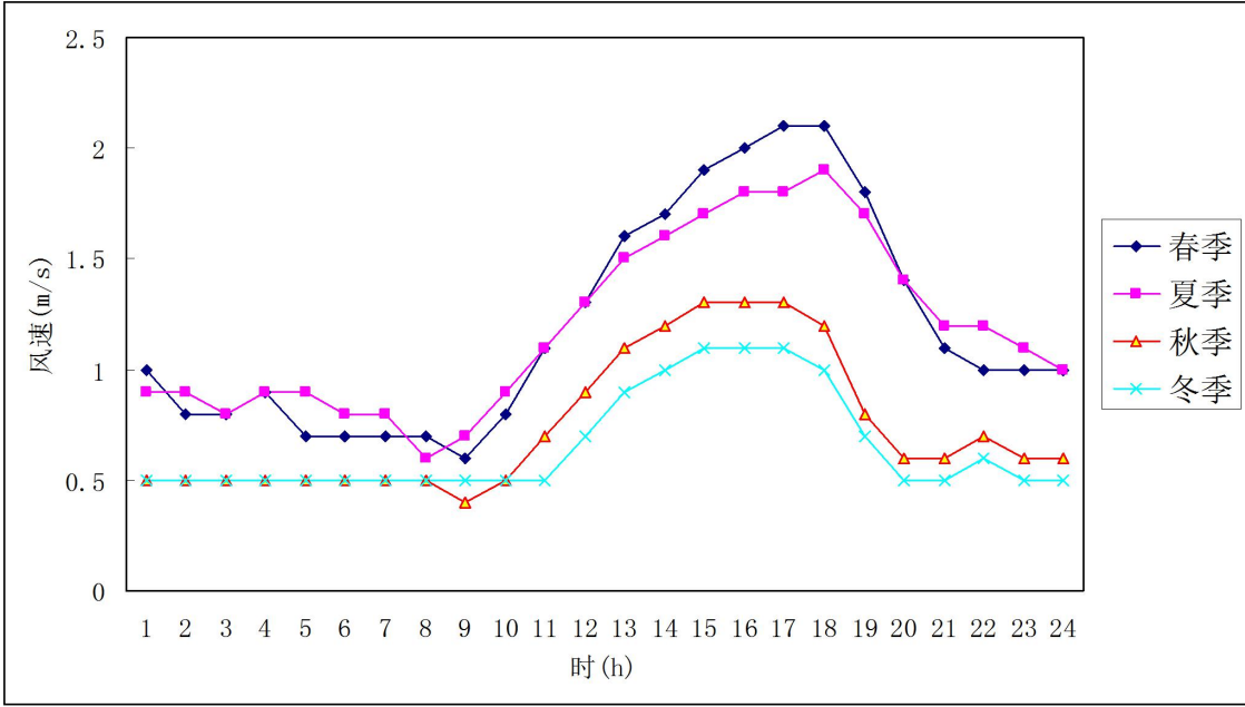
图 5.2-2 季小时平均风速的日变化
