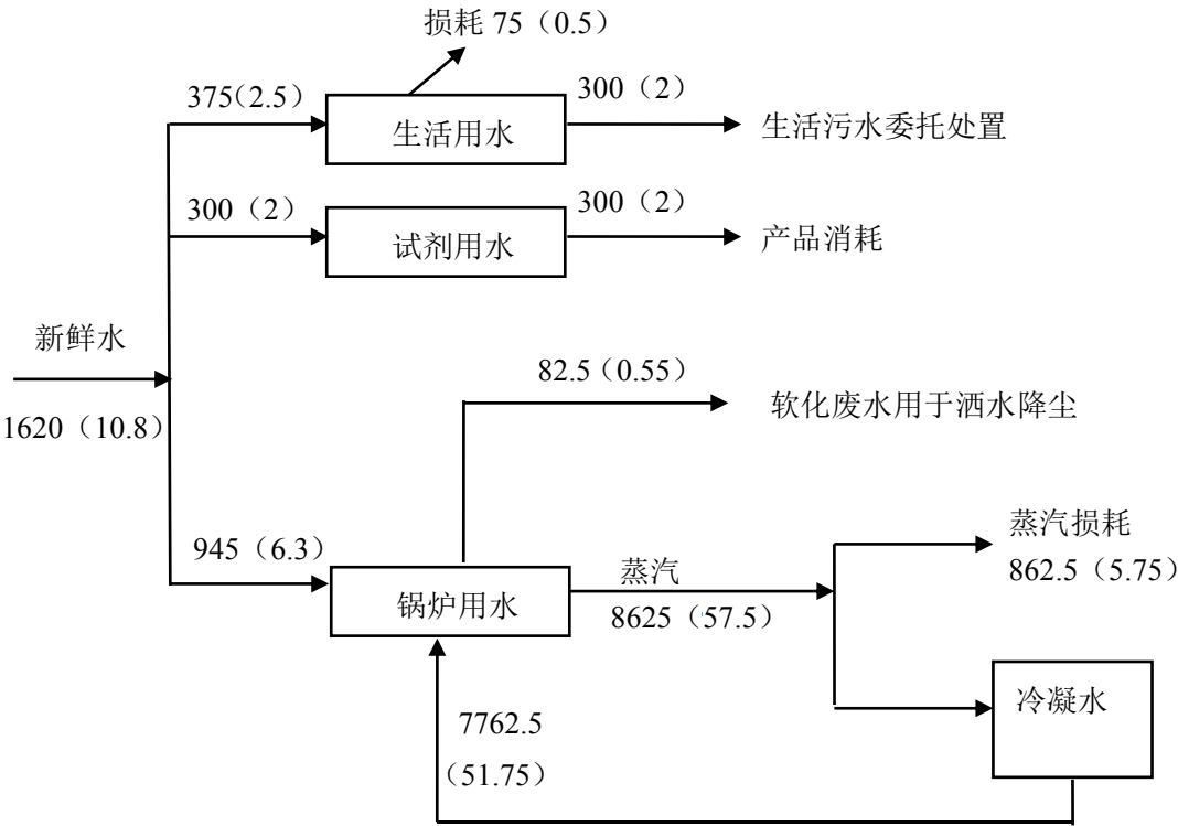
图 3.3-5 项目水衡图（单位：m³/a）
