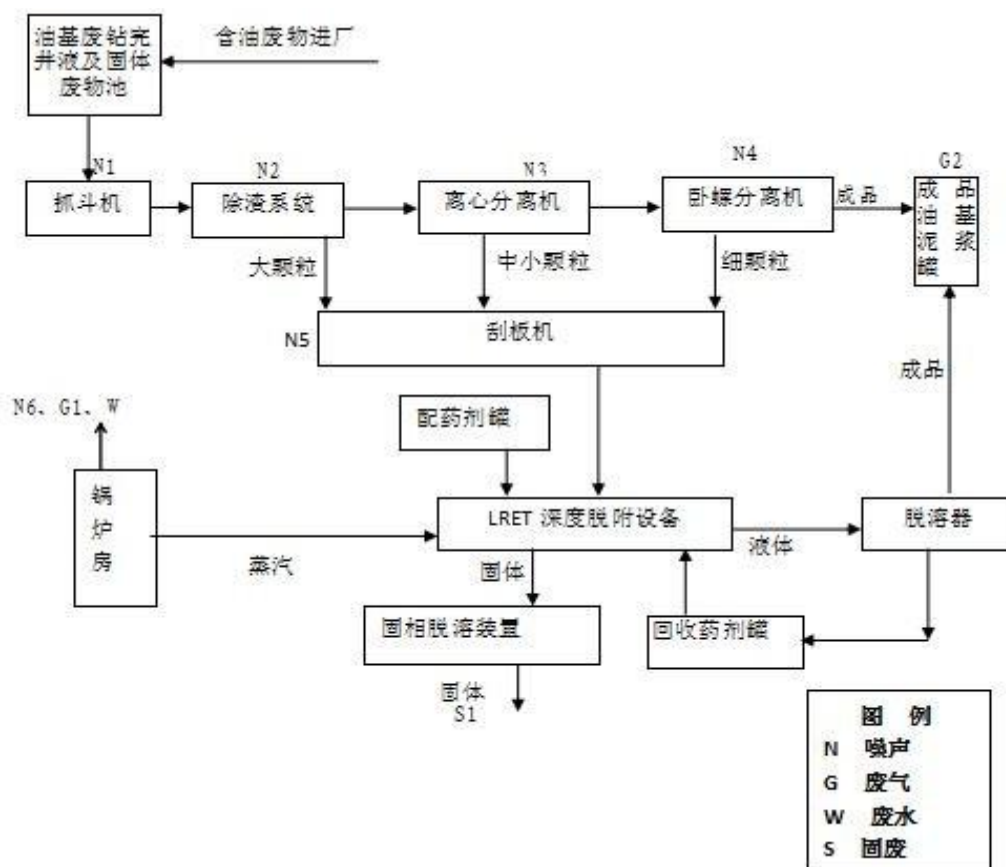
图3.1-2 工艺流程及产污环节示意图
