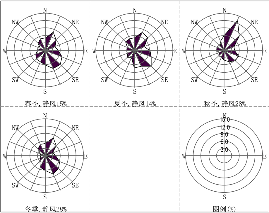
图 5.2-4 拜城县各季风向玫瑰图
