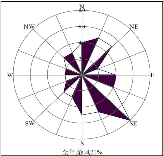
图 5.2-5 拜城县全年风向玫瑰图
