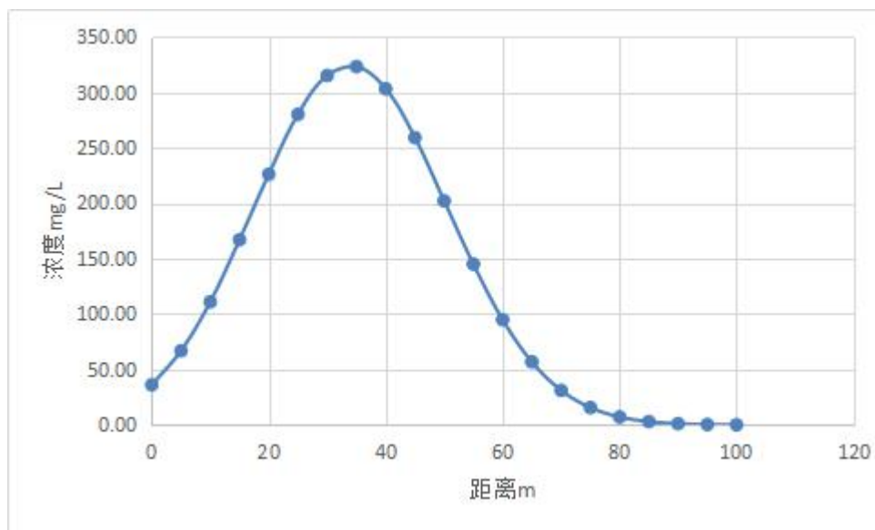
图 5.3-2 污染物 1000 天扩散分布图
