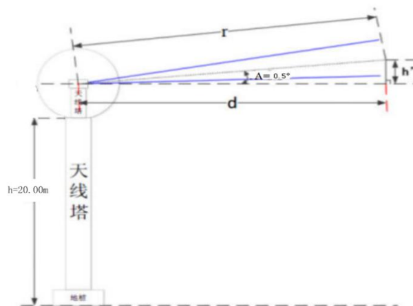
图 4-1 天线前方限高计算示意图
