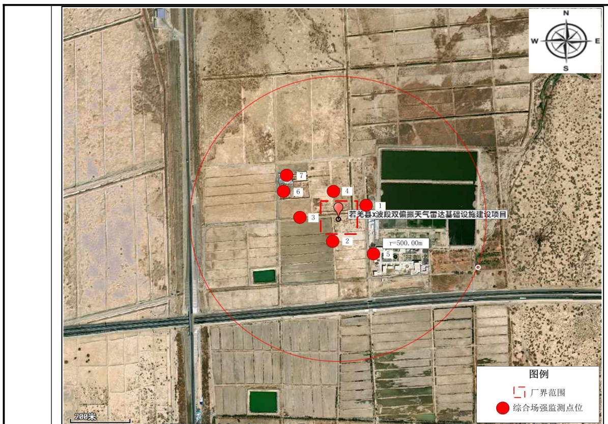
图 3-2 电场强度监测点位图
