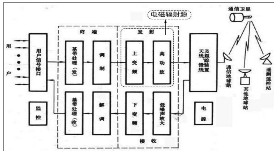
图 2-3 卫星地面站发送传输信号流程示意图
