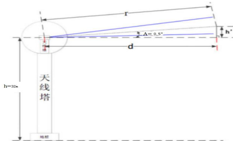
图 4-1 天线前方限高计算示意图
