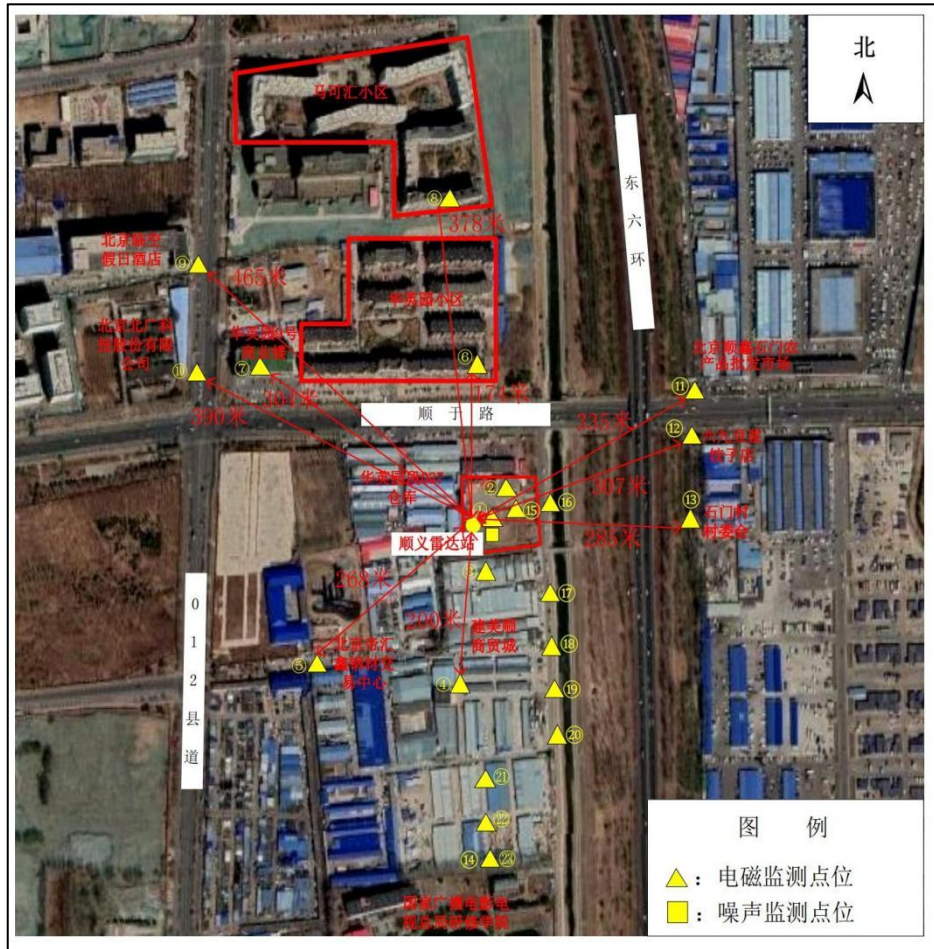
图 4-4 顺义雷达站检测布点图
