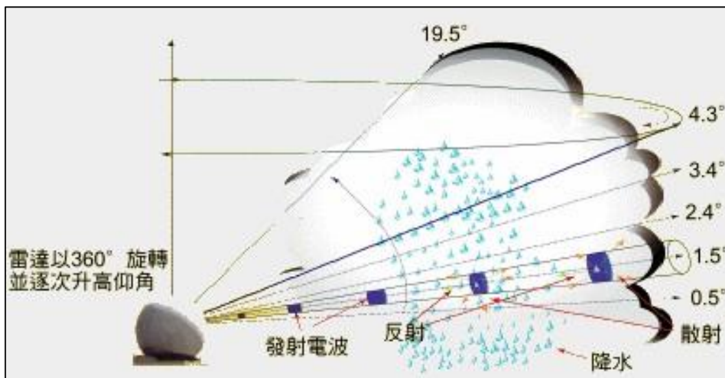
图 2-1 X波段气象雷达系统工作原理图
