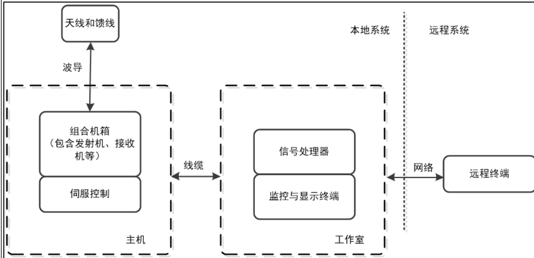
图 2-2 X 波段气象雷达系统组成示意图
