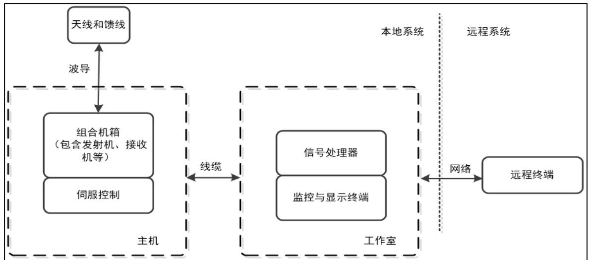
图 2-2 X 波段气象雷达系统组成示意图
