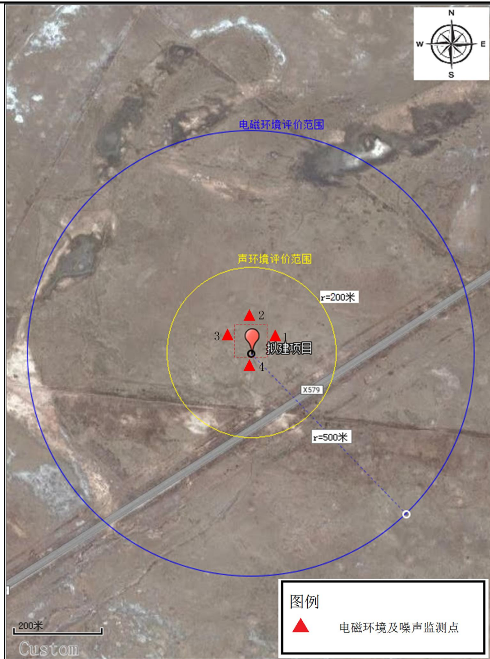
图 3-1 监测点位置示意图
