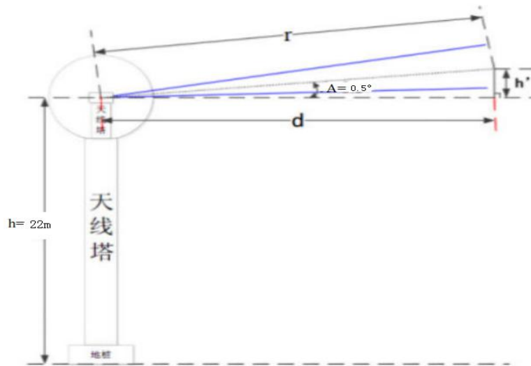
图 4-1 天线前方限高计算示意图
