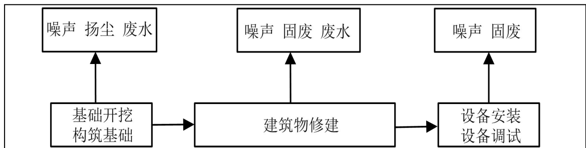
图 2-3 施工期工艺流程及排污节点图
