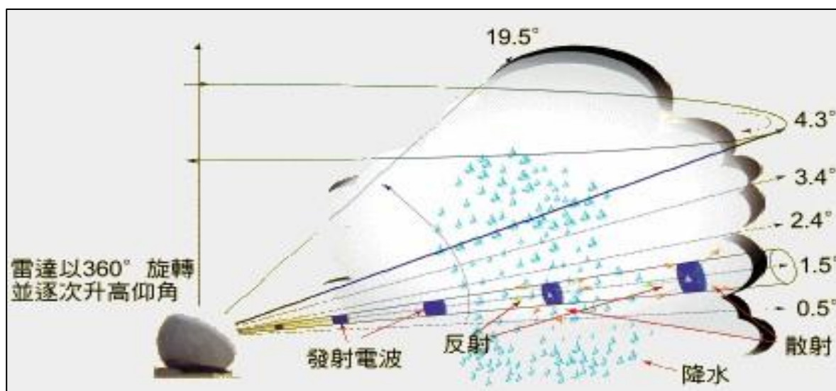
图 2-1 X波段气象雷达系统工作原理图
