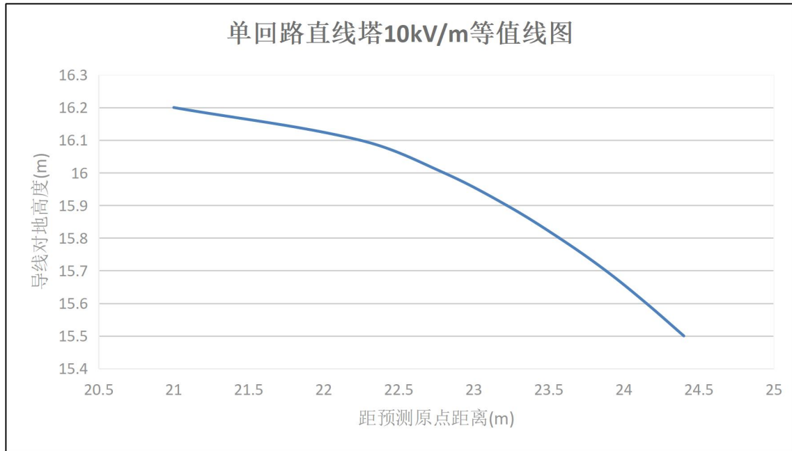
图 6.1-9 单回输电线路 10kV/m 等值线图
