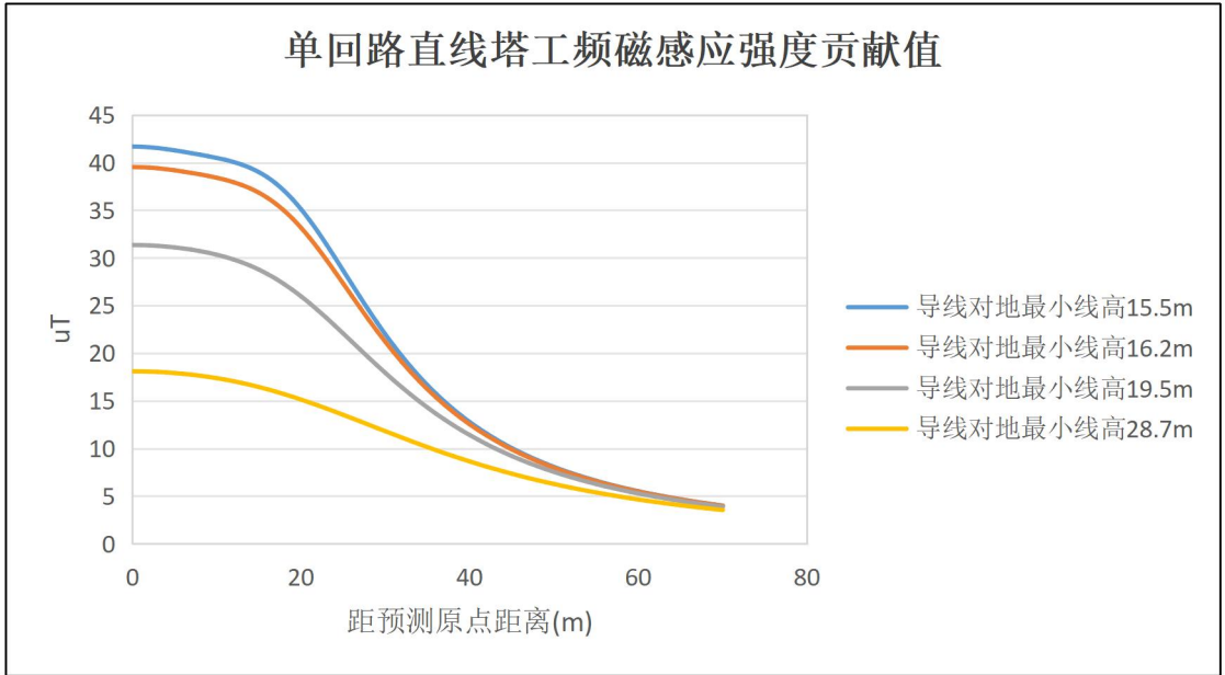
图 6.1-7 单回输电线路工频磁感应强度分布图
