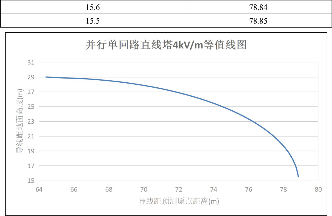
图 6.1-12 并行单回路 4kV/m 等值线图
