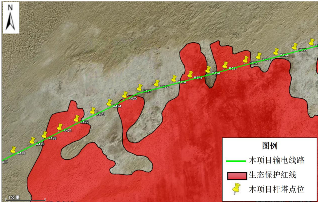
图 7.2-3（续） 38 团规划机场附近线路与红线位置关系图
