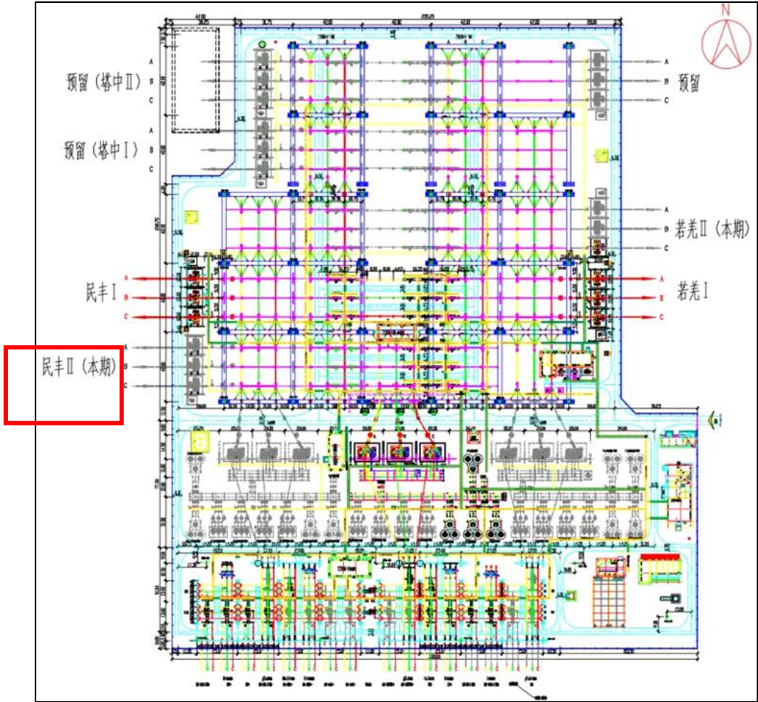
图 3.1-4 且末 750kV 变电站平面布置示意图
