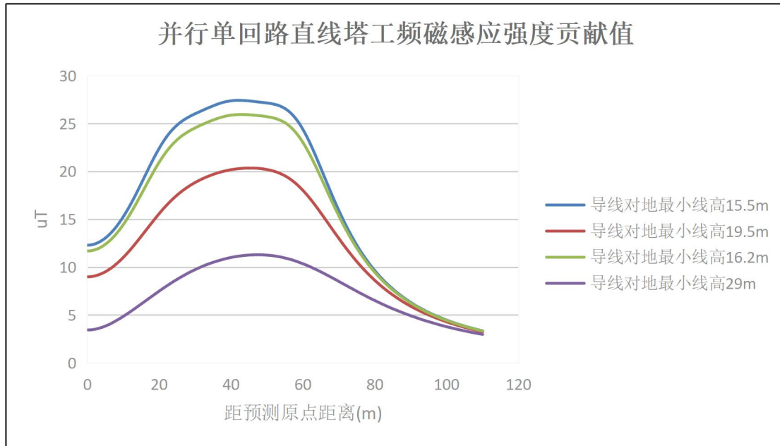
图 6.1-11 并行单回路工频磁感应强度分布图
