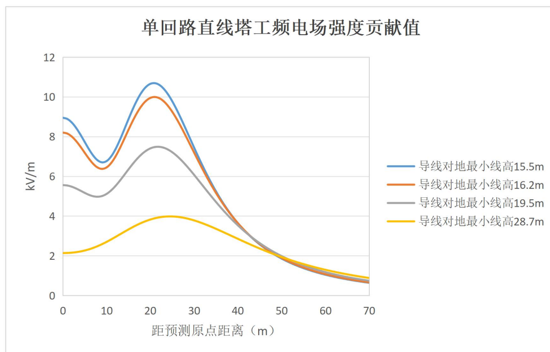
图 6.1-6 单回输电线路工频电场强度分布图
