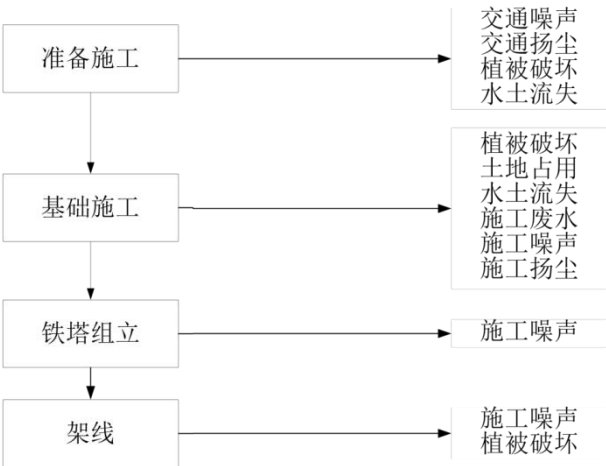
图 3.3-1 输电线路工程施工工艺及产污环节
