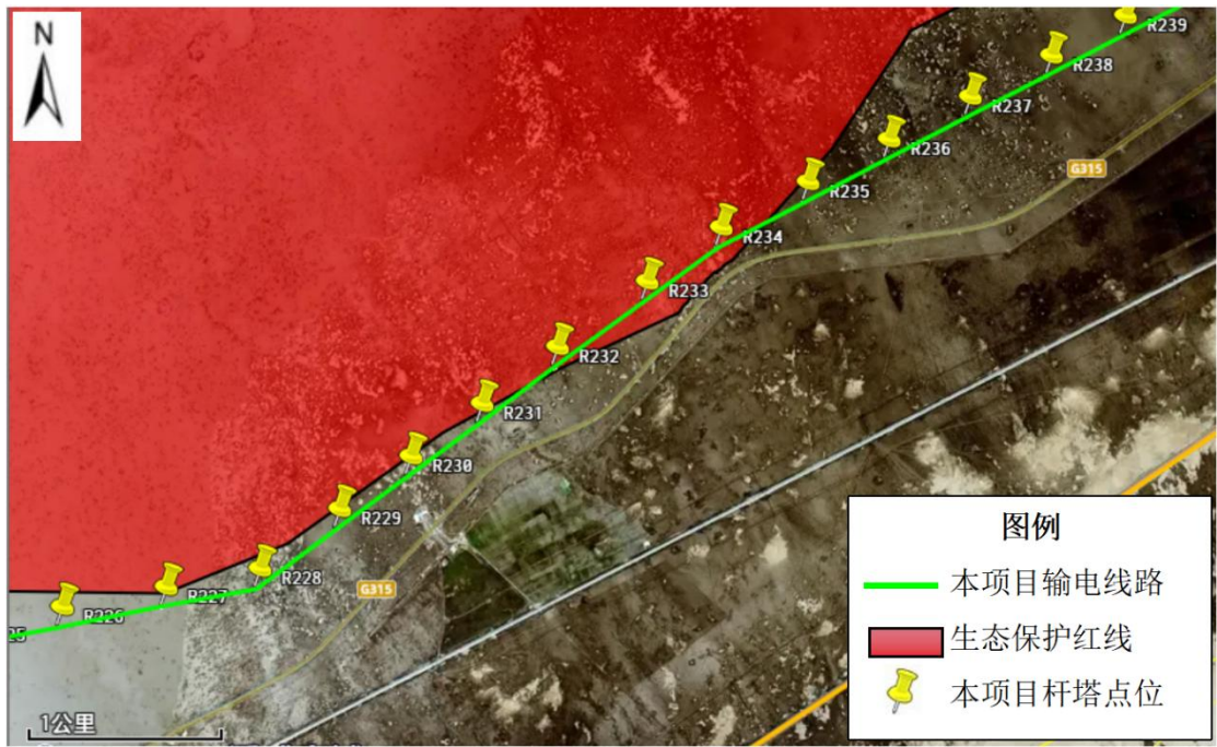
图 7.2-2 牙通古孜河东侧至安迪尔河两侧线路与红线位置关系图
