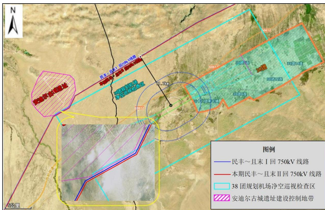
图 3.1-16 本工程路径与规划 38 团机场净空巡视检查区关系图
