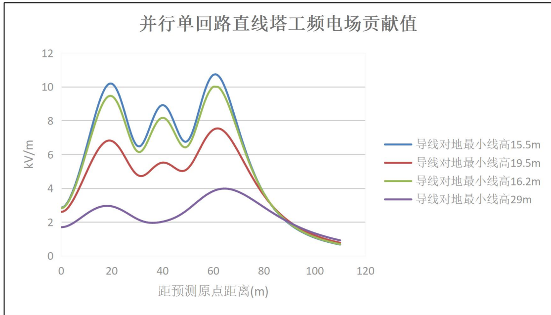
图 6.1-10 并行单回路工频电场强度分布图
