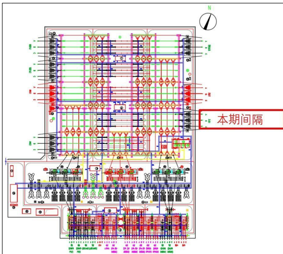
图 3.1-1 民丰 750kV 变电站平面布置示意图
