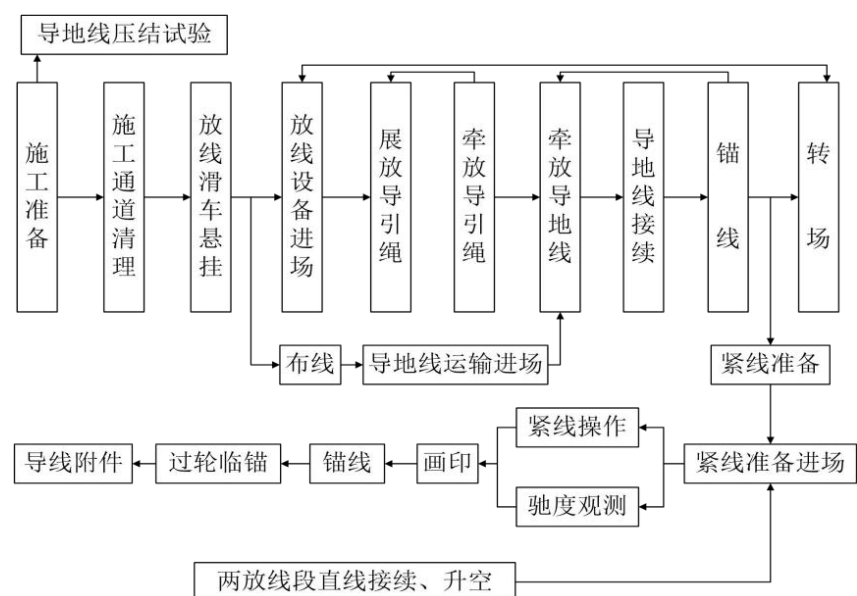
图 3.1-21 架线施工流程图
