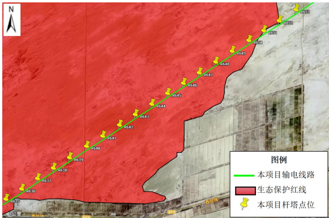
图 7.2-4（续） 且末 750kV 变附近线路与红线位置关系图
