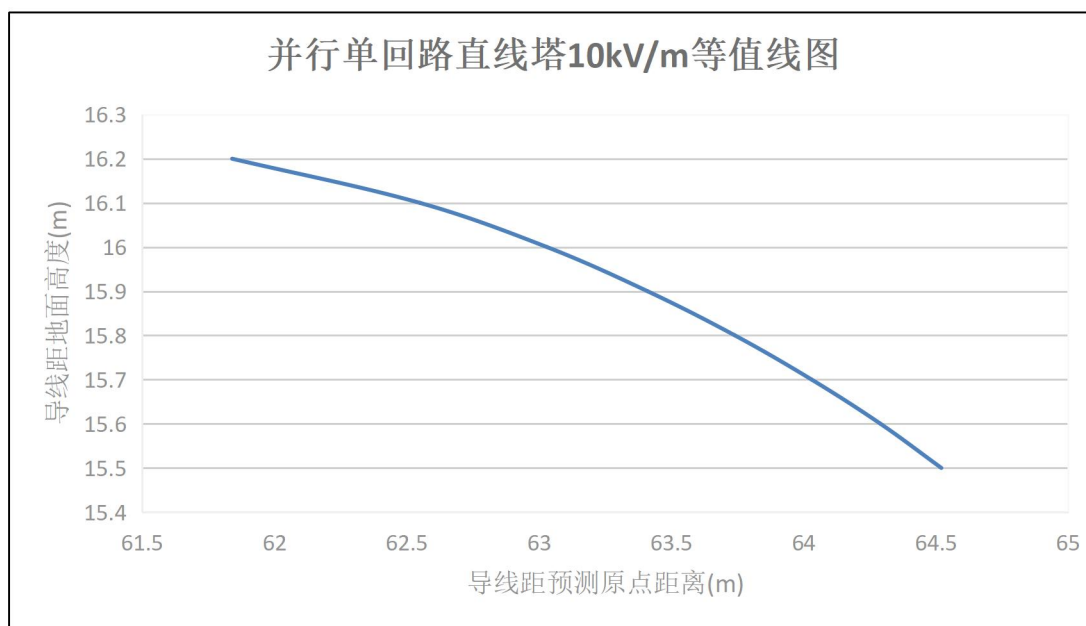
图 6.1-13 并行单回路 10kV/m 等值线图
