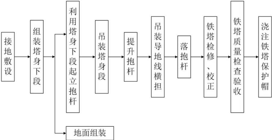
图 3.1-20 铁塔组立接地施工工艺流程图
