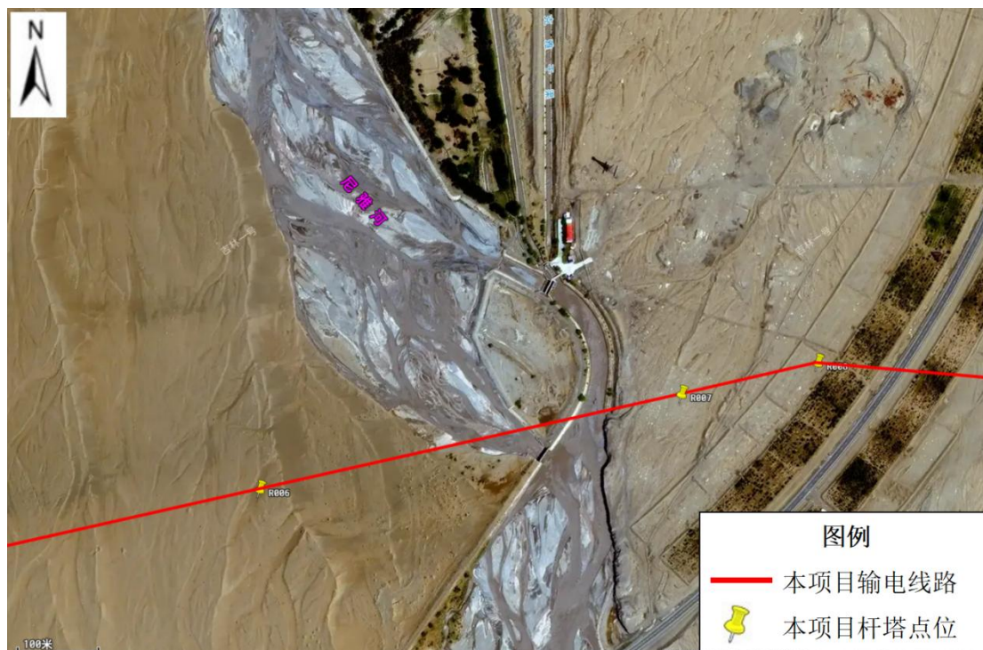
图 4.2-1 线路跨越尼雅河位置示意图
