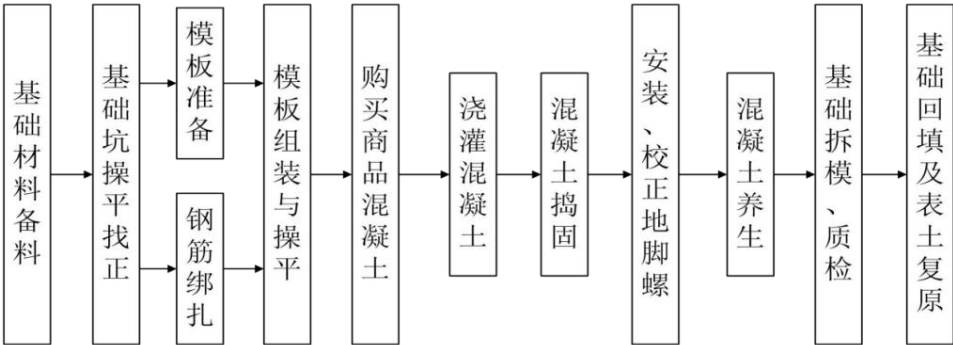
图 3.1-19 基础施工工艺流程图
