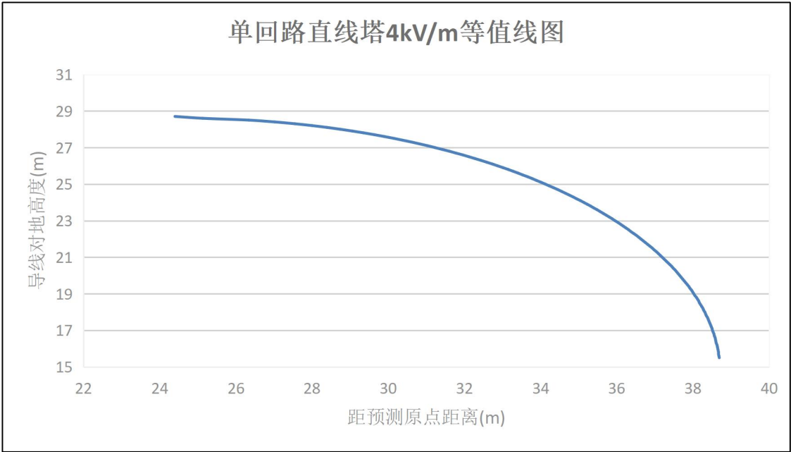
图 6.1-8 单回输电线路 4kV/m 等值线图
