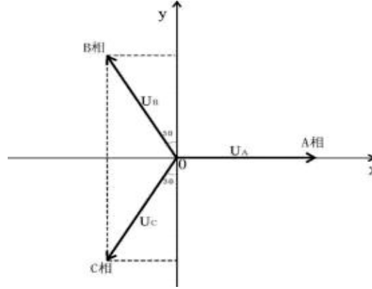
图 6.1-1 对地电压计算图
