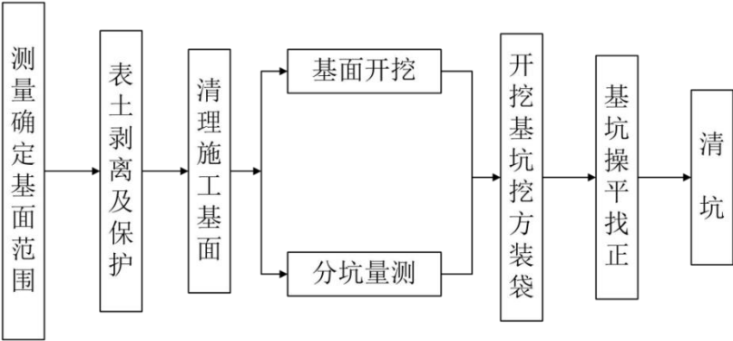
图 3.1-18 基坑开挖施工工艺流程图
