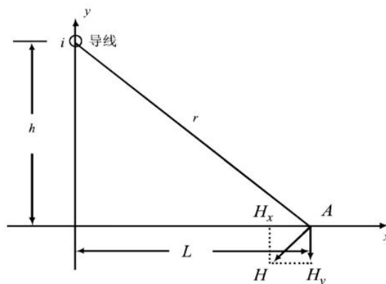
图 6.1-4 磁场向量图
