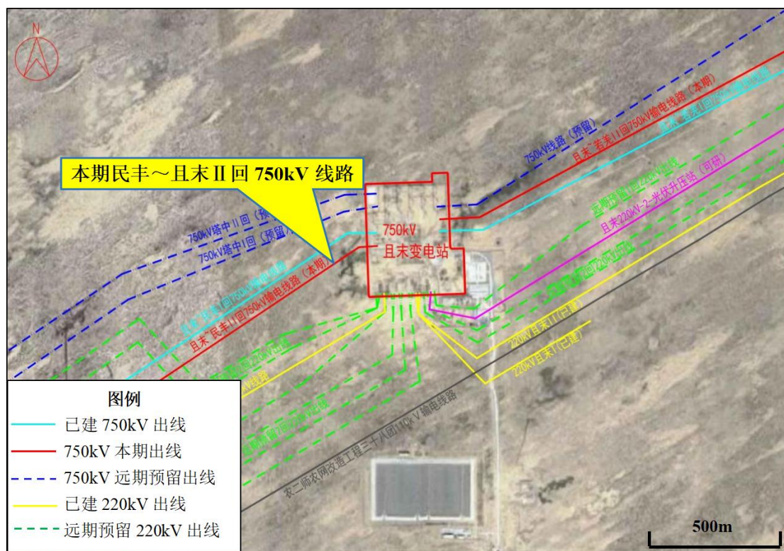
图 3.1-6 且末 750kV 变电站出线规划图
