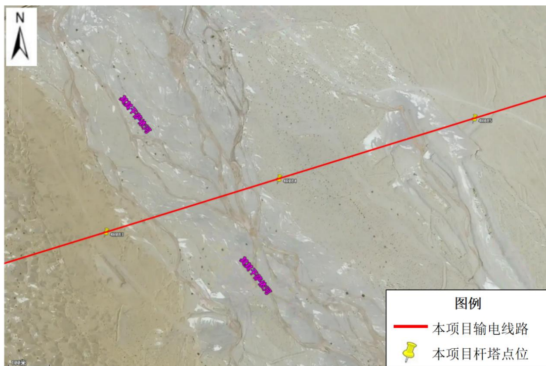
图 4.2-3 线路跨越其其干萨依河位置示意图
