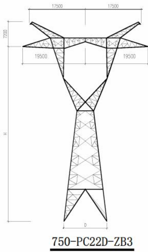
图 6.1-5 本项目输电线路电磁理论预测典型塔型
