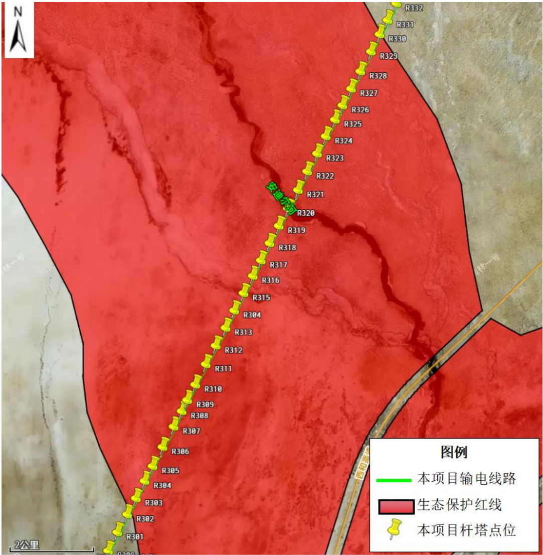
图 7.2-2（续） 牙通古孜河东侧至安迪尔河两侧线路与红线位置关系图
